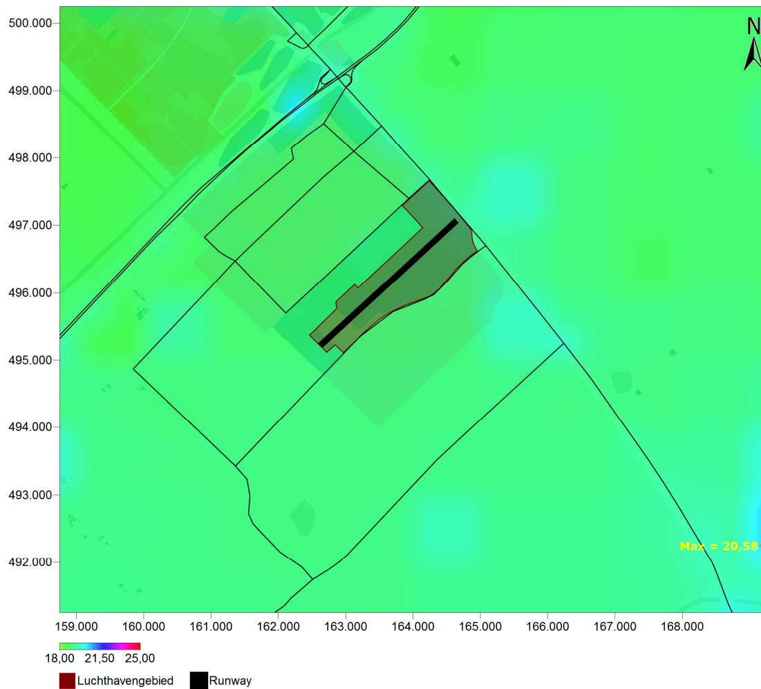
Figuur 31 Resulterende jaargemiddelde concentratie PM 10 [µg/m 3 ] inclusief de voorgenoemde activiteit (45k) in het zichtjaar 2025 inclusief een 3 e aansluiting op de snelweg A6.
