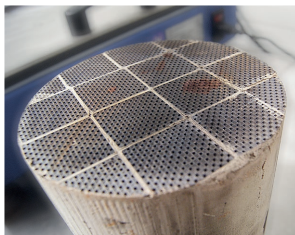
Figuur 5. Ingezoomd beeld van het roetfilter van Figuur 2: de kanalen zijn duidelijk te zien (foto: TNO).
