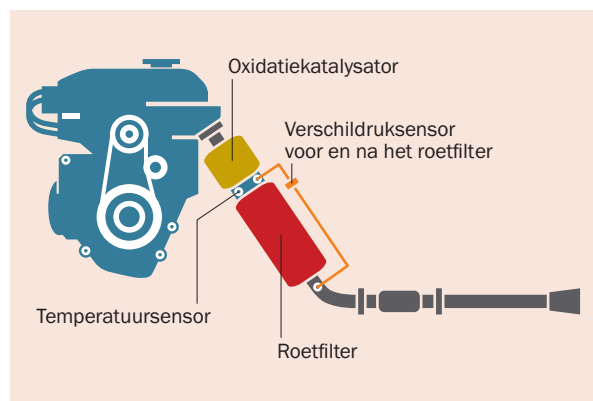
Figuur 4. Het roetfilter bevindt zich achter de motor. In de meeste gevallen zijn auto's met roetfilter ook voorzien van een oxidatiekatalysator, die voor het roetfilter is geplaatst.
