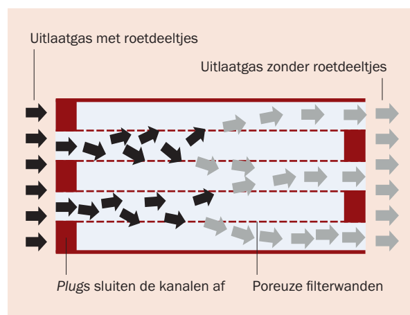
Figuur 6. De schematische tekening laat zien dat een roetfilter is opgebouwd uit vele afgesloten kanalen. Door deze afsluitingen, ook wel plugs genoemd, kunnen de uitlaatgassen alleen door de filterwanden naar buiten stromen. De roetdeeltjes blijven 'plakken' in de filterwand.
