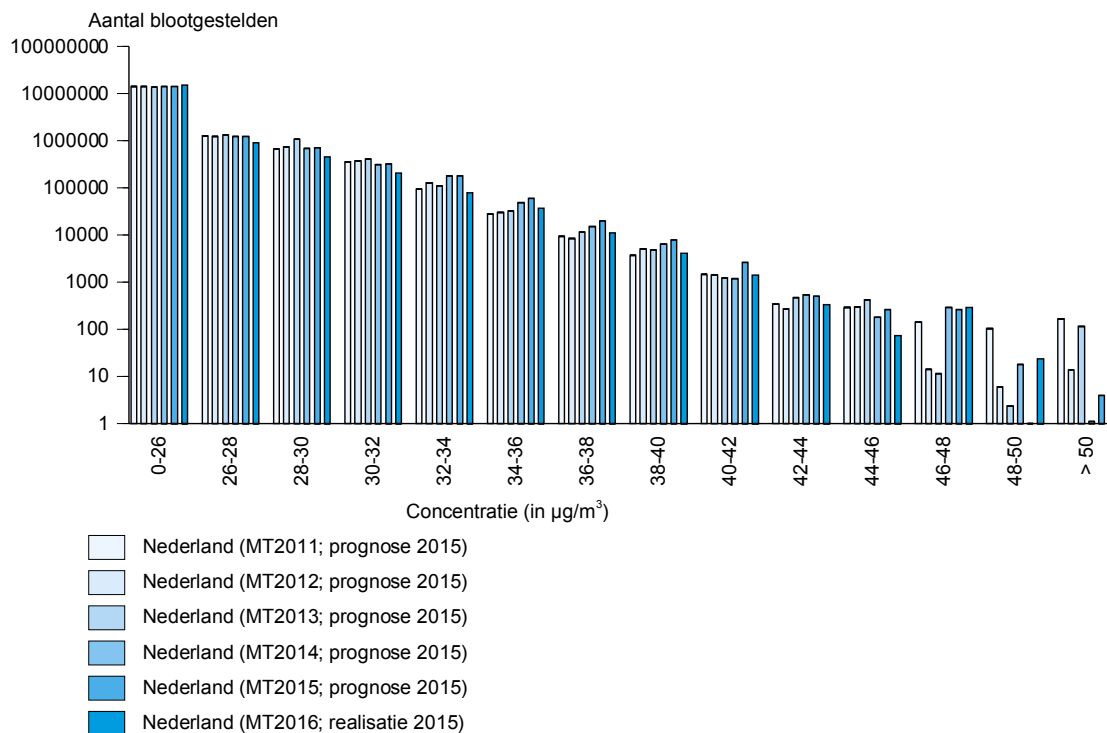
Figuur 17 NO 2 : het aantal mensen dat in 2015 (prognoses en realisatie) aan een bepaalde concentratie wordt blootgesteld in Nederland.
