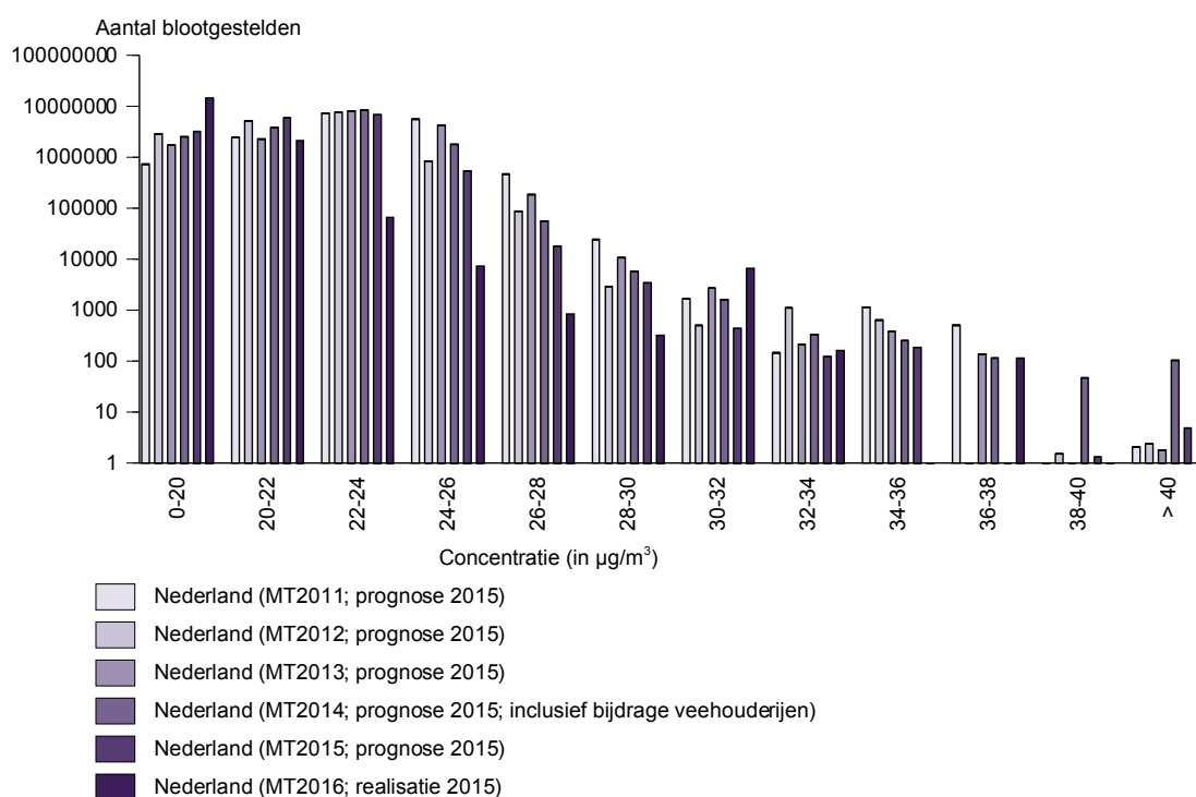
Figuur 18 PM 10 : het aantal mensen dat in 2015 (prognoses en realisatie) aan een bepaalde concentratie wordt blootgesteld in Nederland.
