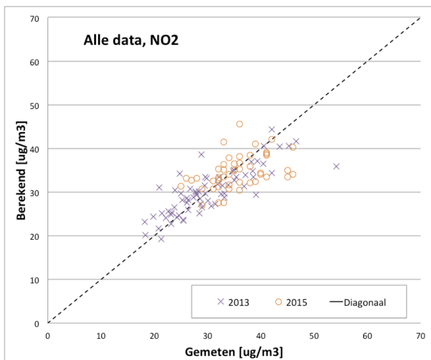
Figuur 22 Gemeten en berekende \text{NO}_2 -concentraties voor 2013 en 2015.
