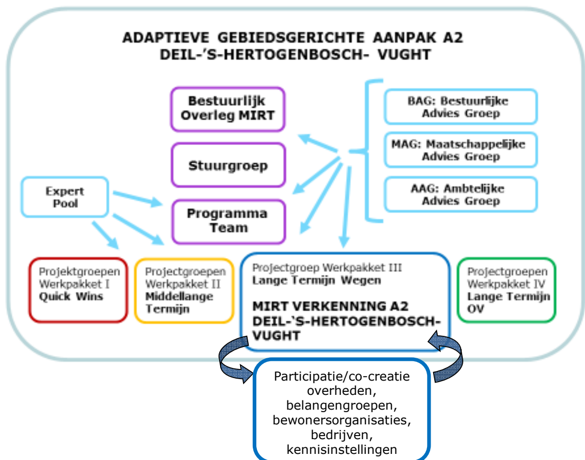
Figuur 5: organisatieschema
