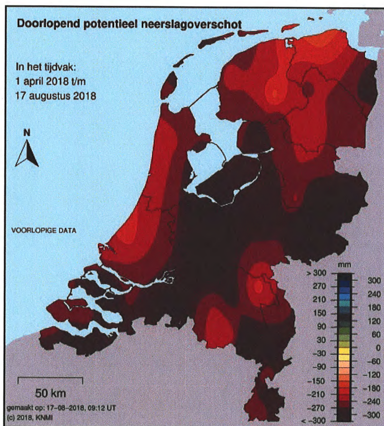
Figuur 1. Ruimtelijke verdeling potentieel neerslagoverschot van 1/4/2018 tot 17/8/2018 (bron: KNMI.nl).
