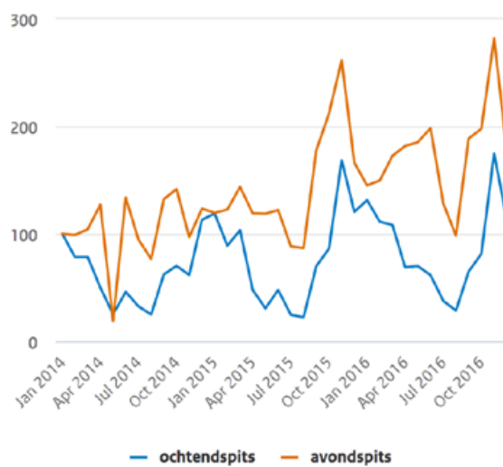
Indicatie van de ontwikkeling van reistijdverlies in ochtend- en avondspits (07.00-09.00 uur; 16.00-18.00 uur) op provinciale en gemeentelijke wegen (links) en op rijkswegen (rechts) in 2014-2016 per maand, op basis van gegevens van INRIX en NDW (kalenderjaar 2014=100). Bron: KiM.
