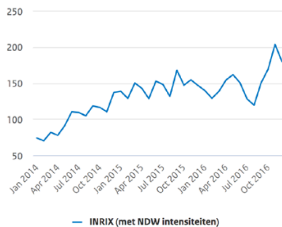
Reistijdverlies op provinciale en doorgaande gemeentelijke wegen
