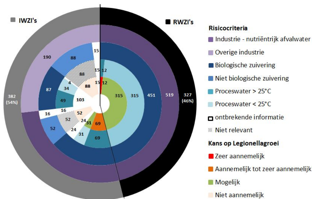
Figuur 4.1. Schematisch overzicht van het aantal AWZI's met bijbehorende risicocriteria en kans op groei van Legionella . In de buitenste schil van de figuur is het aantal AWZI's opgesplitst in 327 RWZI's (zwart) en 382 IWZI's (grijs). De volgende drie schillen geven elk één risicocriterium weer waarin van de RWZI's en IWZI's het aantal installaties aangegeven is voor het type industrie, en daarna het type zuivering en tenslotte de temperatuur van het proceswater. In de binnenste schil is de kans op Legionellagroei weergegeven voor de AWZI's met de bijbehorende risicocriteria.
