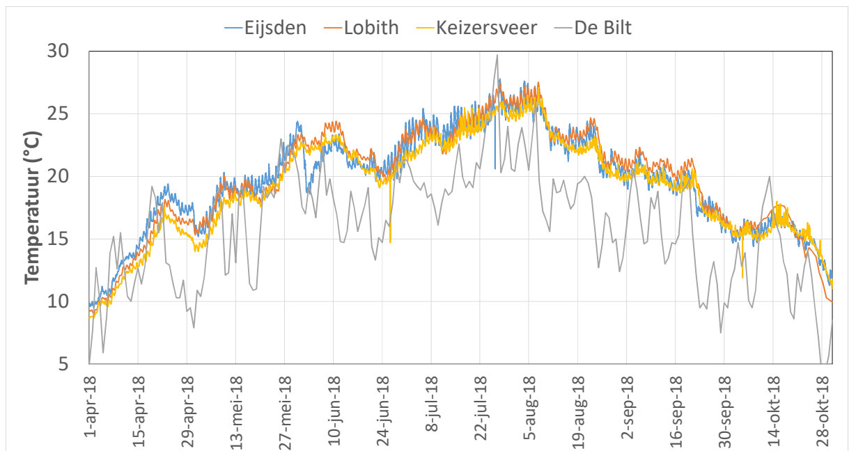
Figuur 3-6. Temperatuur in de periode 1 april 2018 - 31 oktober 2018: oppervlaktewatertemperatuur in de Maas bij Eijsden en in de Rijn bij Lobith, en daggemiddelde luchttemperatuur gemeten in De Bilt. Data: RWS en KNMI (2019).
