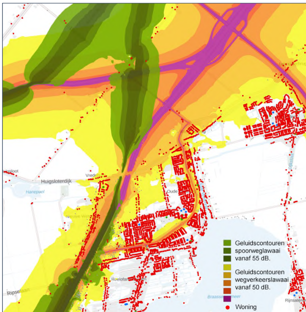
Figuur 8.2: Geluidcontouren spoorweglawaai (groter of gelijk aan 55 dB, groen gekleurd) geprojecteerd op de geluidcontouren van het wegverkeerslawaai (groter of gelijk aan 50 dB, geel/paars gekleurd) van de variant Ringvaartaquaduct Oost
