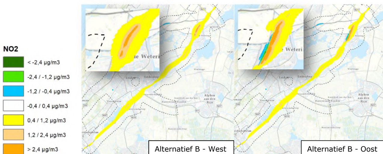
Figuur 8.3: Verschil concentraties stikstofdioxide (NO 2 ) van de alternatieven met uitsneden van de toe- en afnames bij het Ringvaartaquaduct.
