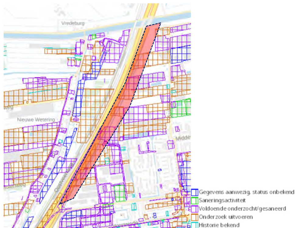
Figuur 9.6: Bodemverontreinigingen bij het nieuw aan te leggen Ringvaartaquaduct in de alternatieven A-O en B-O. Het zoekgebied voor de nieuwe wegligging is met rood weergegeven.
