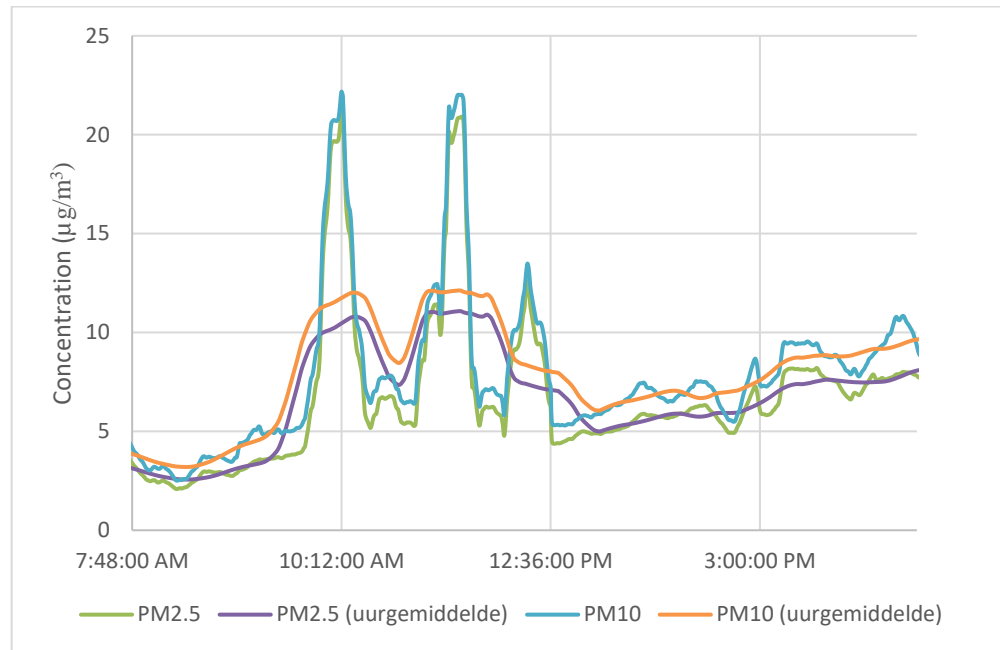
Figuur 6: Meting van fijnstof met behulp van een FIDAS. Om 9.45u (UTC) is de kachel opgestart en er is daarna onafgebroken gestookt. De groene lijn (PM 2.5 ) en de blauwe lijn (PM 10 ) representeren de hoge resolutie meetdata. De paarse lijn (PM 2.5 ) en oranje lijn (PM 10 ) representeren het lopende gemiddelde over 1 uur. Vanaf circa 13.15u is de meetwagen verplaatst.
