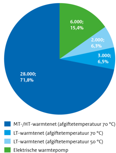
Figuur 6-4: Verdeling woningen naar aardgasvrije warmtebron (DAEB + niet-DAEB), 2020 t/m 2050; bron: ABF
