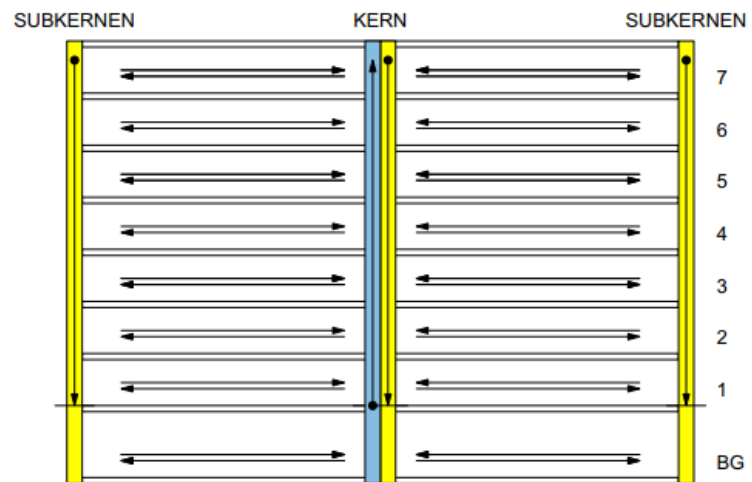
GEBOUW SCHEMA PRINCIPE TRAPPEN
