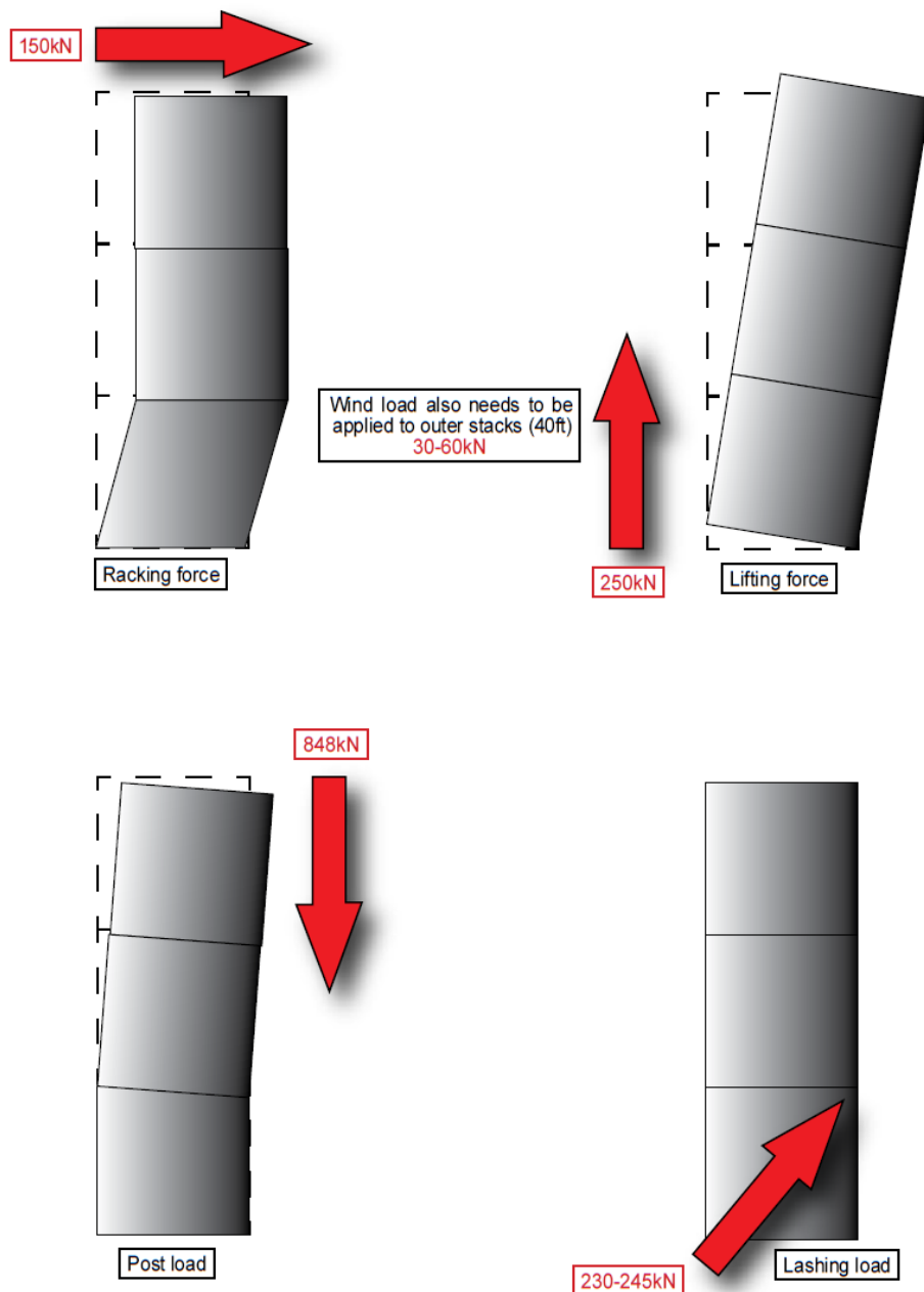
Afbeelding 12: Maximale krachten op containers [6].
