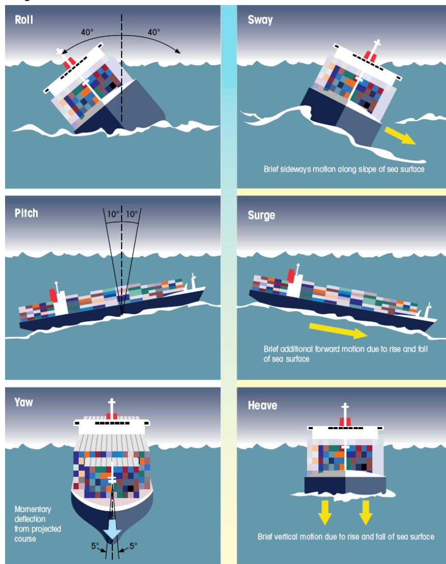
Afbeelding 11: Scheepsbewegingen containerschip [6]
