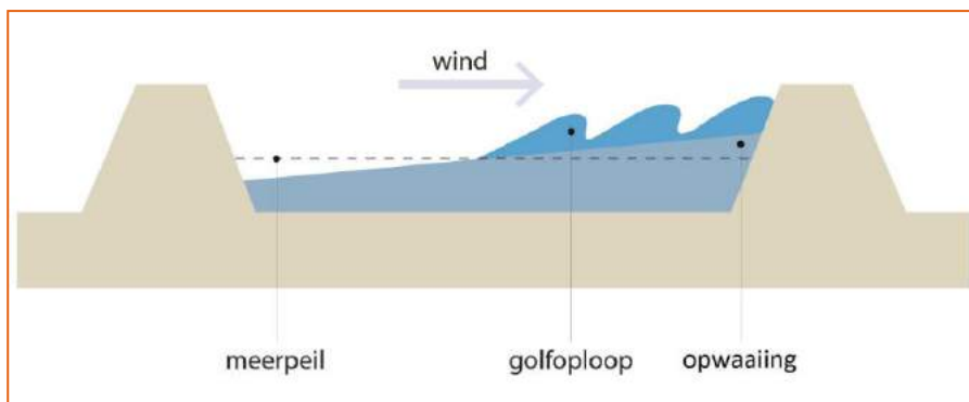
Figuur 3-1 Schematische weergave van meerpeil, golfploop en opwaaiing 3
