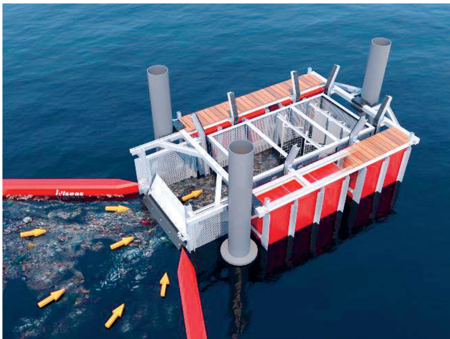
Figuur 5-c. Prototype plastic vang in de Vijfsluizerhaven, Nieuw Maas.
