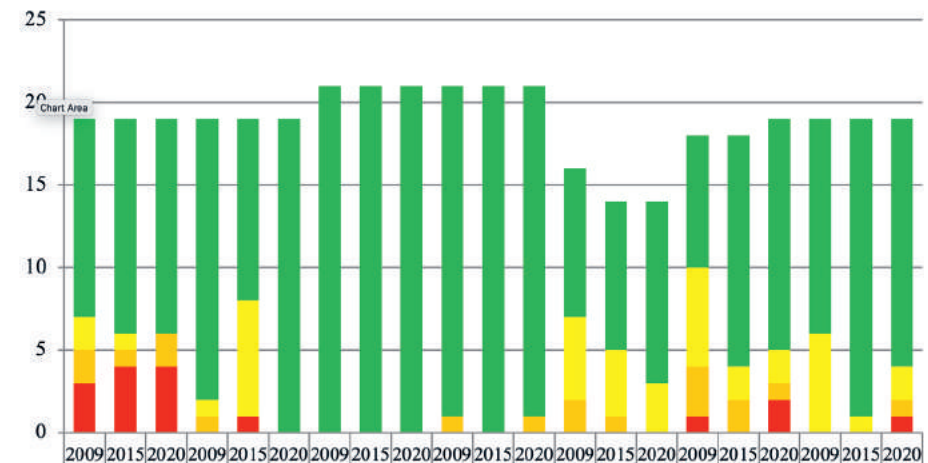
Figuur 3-p. Beoordeling van de fysisch-chemische parameters in het oppervlaktewater voor het stroomgebied Rijn in 2009, 2015 en 2021 (aantal waterlichamen; groen = (zeer) goed, geel = matig, oranje = ontoereikend, rood = slecht).
