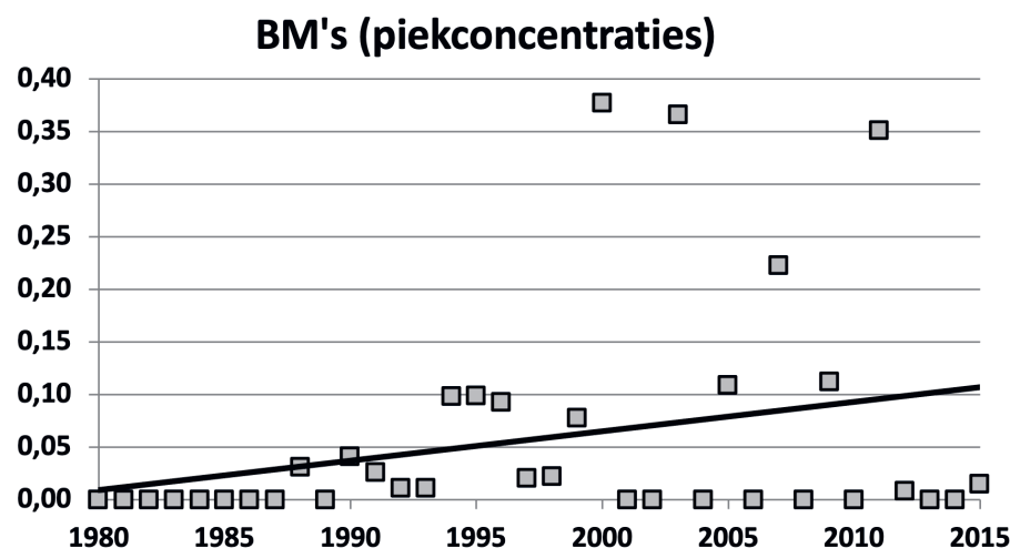
Figuur 5-d. Verloop van de toxische druk door een mengsel van bestrijdingsmiddelen in de Dommel, bepaald met de Ecologische SleutelFactor Toxiciteit (RIVM in samenwerking met waterschap De Dommel).
