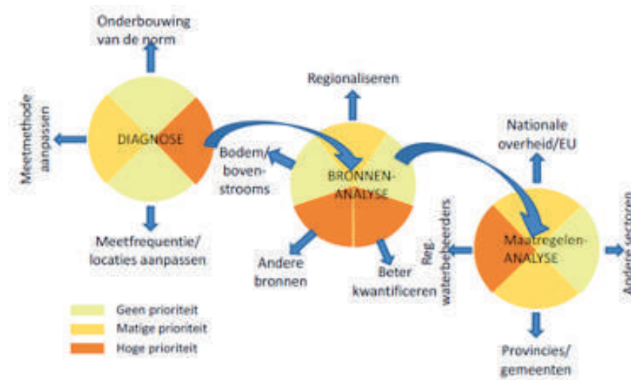
Figuur 4-a. Werkwijze bij het onderzoek naar het probleem (diagnose: circa 60 stoffen), de oorzaak (bronnenanalyse: circa 25 stoffen) en mogelijke maatregelen (maatregelenanalyse: 15 stoffen) voor chemische stoffen die regelmatig milieukwaliteitseisen overschrijden.
