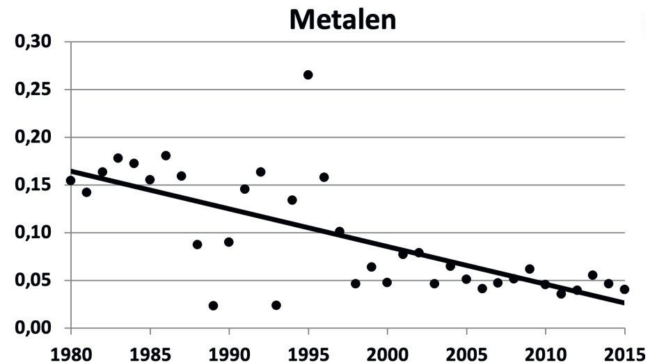
Figuur 5-c. Verloop van de toxische druk door een mengsel van metalen in de Dommel, bepaald met de Ecologische Sleutelfactor Toxiciteit (RIVM in samenwerking met waterschap De Dommel).
