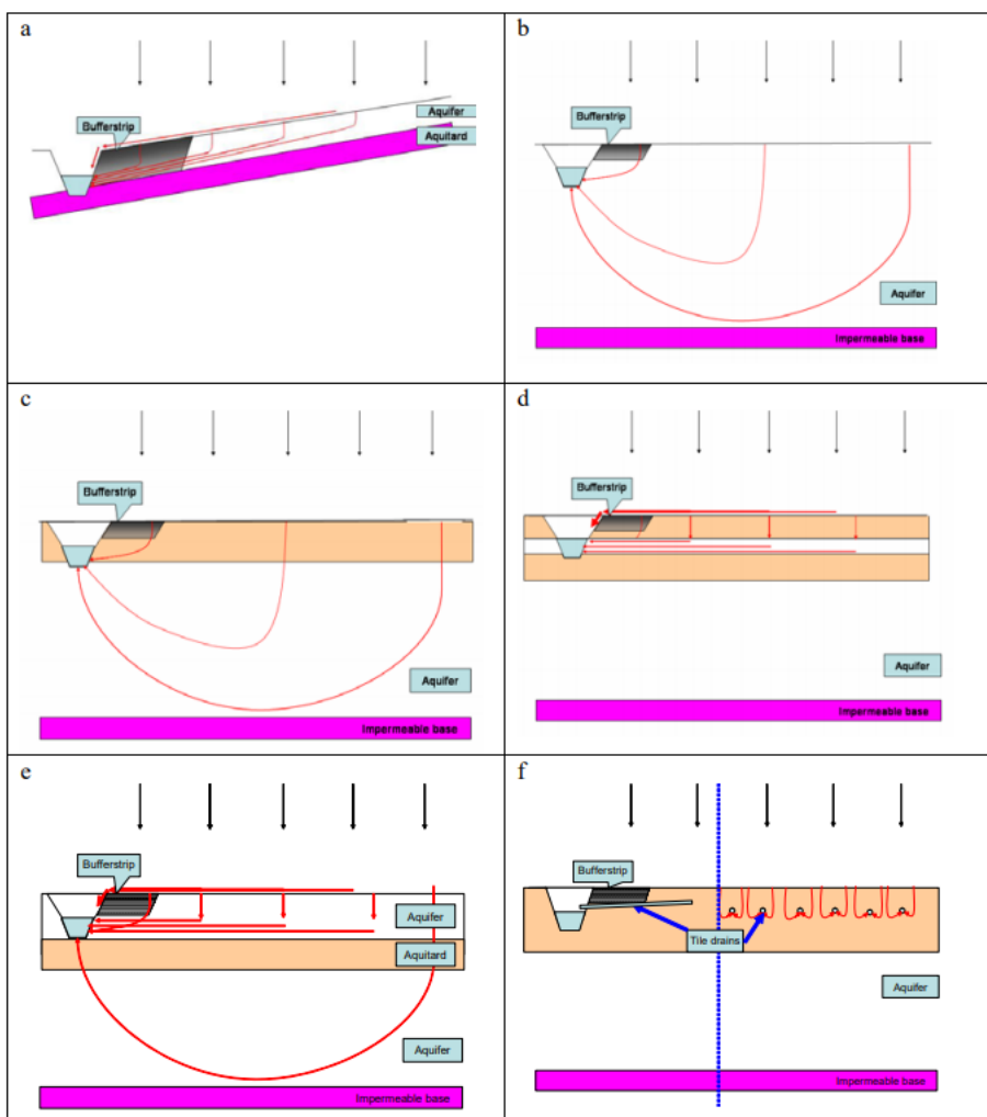
Figuur B6.1.1. Schematische weergave van zes onderscheiden geohydrologische profielen voor het karakteriseren van grondwaterstroming nabij en onder bemestingsvrije perceelsranden (Bron: Van Bakel et al, 2007)
