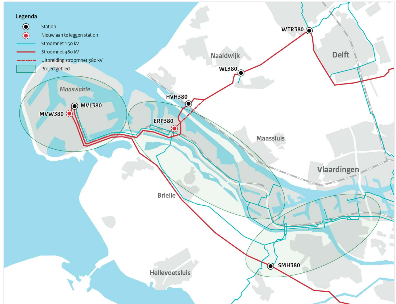
Uitsnede netkaart en gebied voor projecten voor verzwaring elektriciteitsnet Rotterdam-Moerdijk. Alle stroomnetten bestaan uit dubbele circuits.
