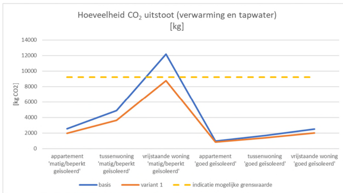
Grafiek 8: CO 2 -uitstoot verwarming en warm tapwater [kg]: basissituatie en variant 1 (hybride warmtepomp)
