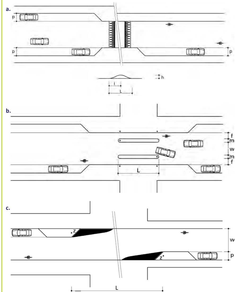
Afbeelding 4.3. Snelheidsremmers op erftoegangswegen binnen de bebouwde kom volgens ASVV 11.2.21, 11.2.24, 11.2.25 (CROW, 2021)
