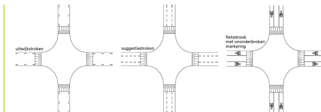
Afbeelding 4.7. Kruispuntplateau ETW60-ETW60 volgens HWO (CROW, 2013a)
