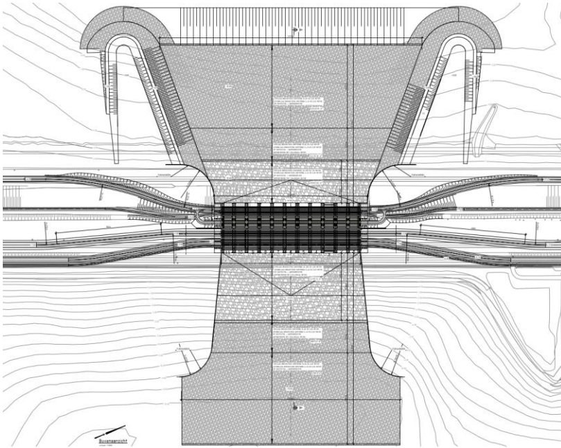
Figuur 6.6: Bovenaanzicht doorlaatmiddel TF-VKA (getijdevariant B2) (bovenzijde is Noordzeezijde, onderzijde is Grevelingenzijde)
