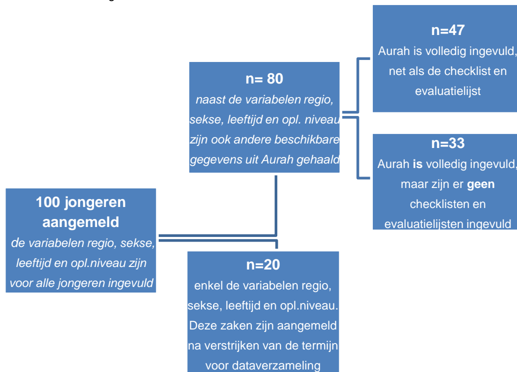
Figuur 1: dataverzameling
