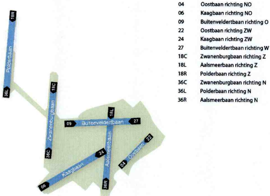
Figuur 2-7 Banenstelsel Schiphol
