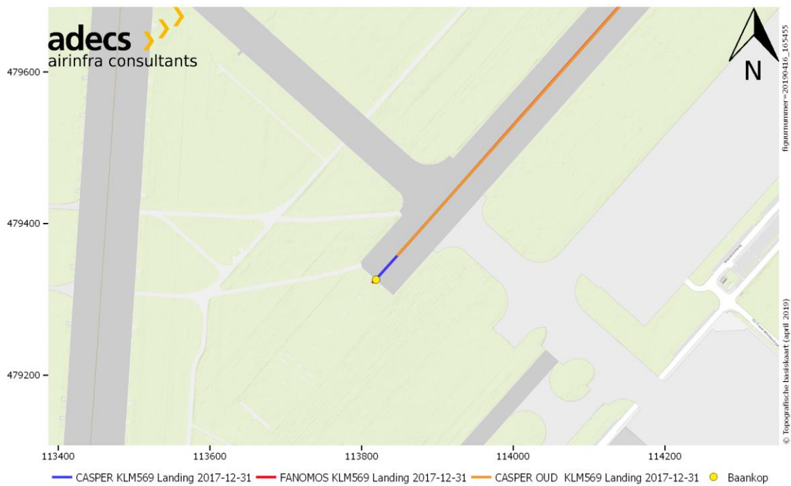
Figuur 4 Vergelijking tussen radartrack van een landing CASPER oud, CASPER en FANOMOS i.c.m. baankop.
