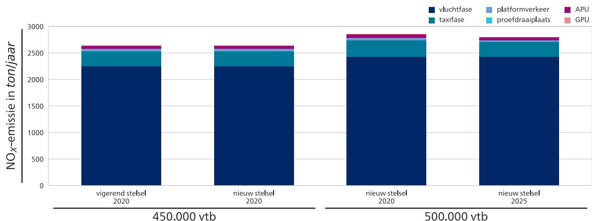
Figuur 7.5 NO x -emissies in tonnen per jaar van de verschillende luchtvaartgebonden bronnen voor de beschouwde situaties. De bijdrage van de vlucht- en taxifase bedraagt steeds ca. 96% van de emissies
