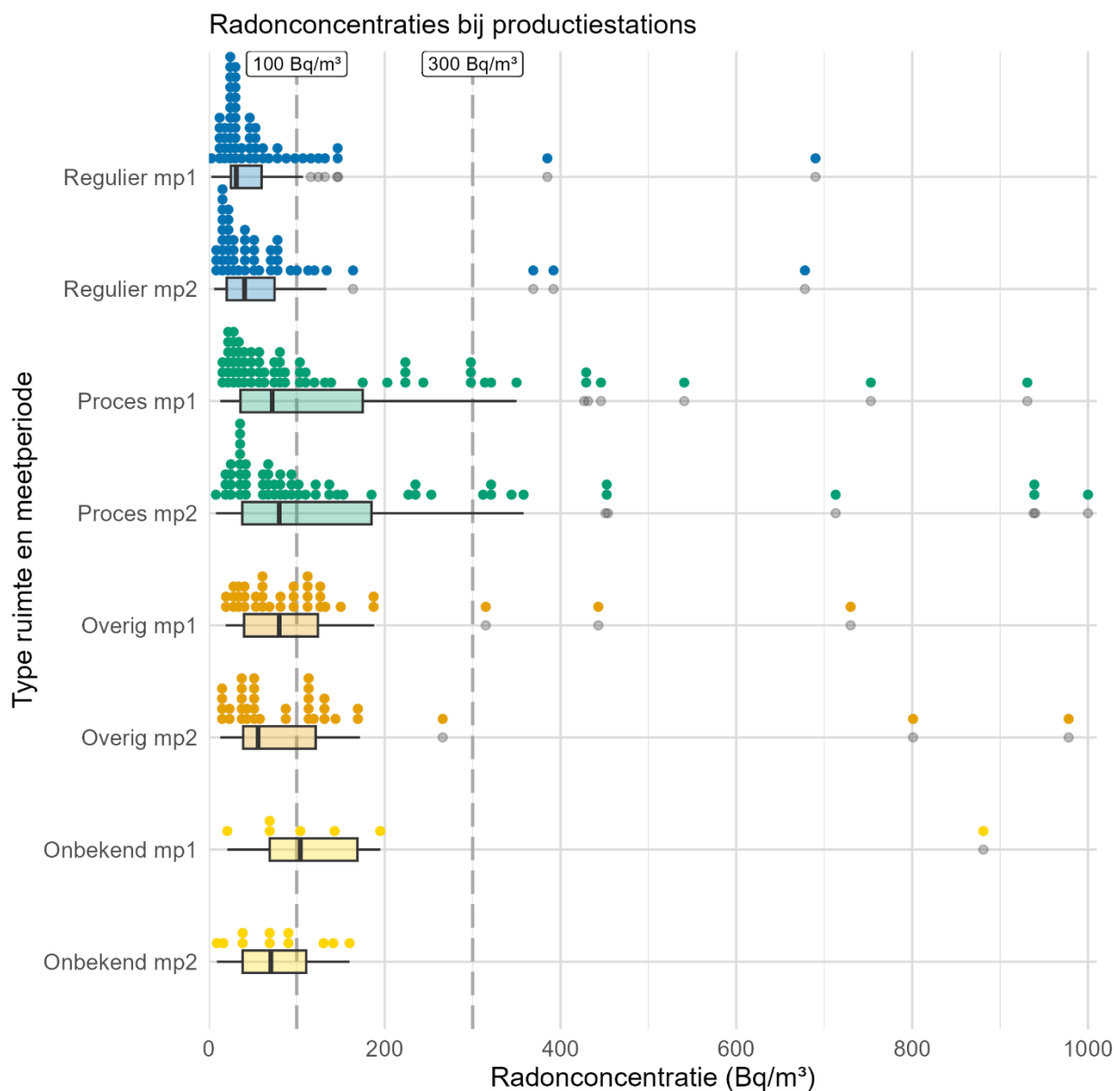
Figuur 10.1 Boxplots en cloudplots van de passieve radonmetingen in verschillende ruimtes bij de productiestations per meetperiode. Bij de cloudplots geeft iedere punt een meetwaarde weer. Bij de boxplots geven de linker- en rechterkant van de box het 25 e en 75 e percentiel weer (de interkwartielafstand), de verticale lijn in de box is de mediaan. De horizontale lijnen ('whiskers') geven aan welke waarden binnen 1,5 keer de interkwartielafstand liggen. Ook weergegeven in de figuur zijn het Nederlandse en maximale Europese referentieniveau (100 en 300 Bq/m³). Meetperiode 1 (mp1) correspondeert ruwweg met de herfst/winter en meetperiode 2 (mp2) met de lente/zomer. Een omschrijving van de indeling van de type ruimtes staat beschreven in paragraaf 10.3.2. De -as is afgekapt op 1000 Bq/m³, 20 meetpunten zijn niet weergegeven. Het gaat om 9 metingen in procesruimtes in meetperiode 1, 6 metingen in procesruimtes in meetperiode 2, 3 metingen in overige ruimtes in meetperiode 1 en 2 metingen in overige ruimtes in meetperiode 2.
