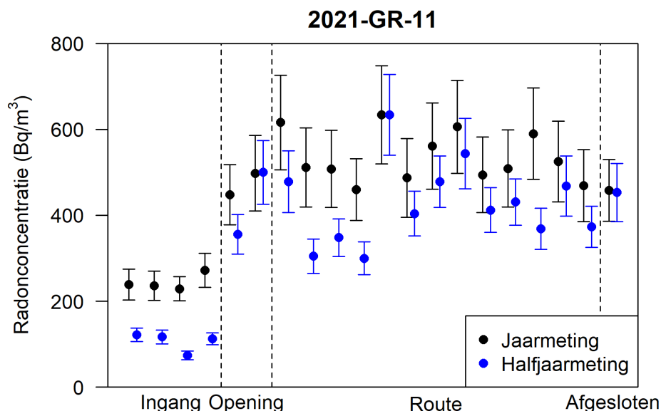
Figuur 6.2 De radonconcentratie in groeve 2021-GR-11, voor vier verschillende categorieën locaties (van links naar rechts): in de buurt van de (hoofd)ingang, bij een ander soort opening (nooduitgang, ventilatieschacht), aan de route, of in een afgesloten (afgesloten, ingestort of doodlopend) deel van de groeve. Meer informatie over de locatieomschrijvingen is te vinden in bijlage 15. Resultaten van de jaar- en halfjaarmetingen op dezelfde locatie zijn naast elkaar geplot. De foutbalken zijn 2 keer de standaarddeviatie van de meting.
