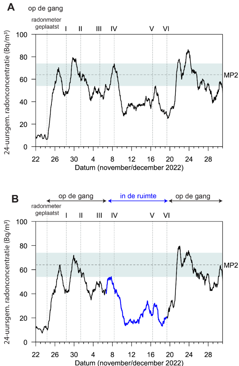
Figuur 10.3 De radonconcentratie gemeten tijdens het reinigen van de nafilterruidtes (tweede set continue metingen). Figuur A geeft de radonconcentratie weer op de gang vlak buiten één van de ruimtes, en figuur B de radonconcentratie die verderop in de gang is gemeten. Een deel van de tijd was de radonmeter in de ruimte zelf geplaatst; dit is weergegeven in blauw. Zes tijden zijn gemarkeerd met verticale stippellijnen: (I) voorbereidingen voor het verwijderen van het oude filtergrind; (II) start verwijderen van het oude filtergrind en schoonmaken van de ruimte (dit duurt drie werkdagen); (III) start schoonmaken van de stenen van het luchtnet en testen van het luchtnet (dit duurt twee werkdagen); (IV) inbrengen van vier lagen nieuw filtergrind gevolg door een week zonder werkzaamheden; (V) inbrengen van nog twee lagen nieuw filtergrind; en (VI) filter op inloop. Daarnaast is een radonconcentratie gemarkeerd: MP2, het resultaat van passieve radonmetingen in een vergelijkbaar filtergebouw tijdens de tweede meetperiode. Het gekleurde horizontale vlak geeft de onzekerheid weer (2 standaarddeviaties) van de passieve meting.
