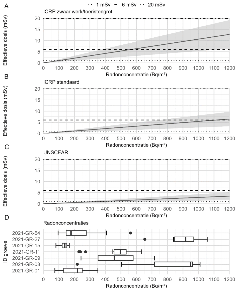
Figuur 15.7 Figuren A-C tonen de effectieve dosis als functie van de radonconcentratie bij een werktijd van 800 uur (95% van de werknemers werken minder dan 800 uur per jaar in de groeve). Er is gerekend met de DCC van de ICRP voor zware werkzaamheden/werkzaamheden in een toeristengrot (A), de DCC van de ICRP voor standaard werkzaamheden (B) en de DCC van UNSCEAR (C). Het grijze vlak geeft de variatie in evenwichtsfactor aan. Voor de variatie van de evenwichtsfactor is gerekend met een F van 0,2 tot 0,6. Voor de lijnen is gerekend met een meest waarschijnlijke waarde voor F , namelijk 0,4. Het onderste deel van de figuur (D) geeft de jaargemiddelde radonconcentraties in de deelnemende groeven (voor uitleg over de boxplots, zie Figuur 6.1).
