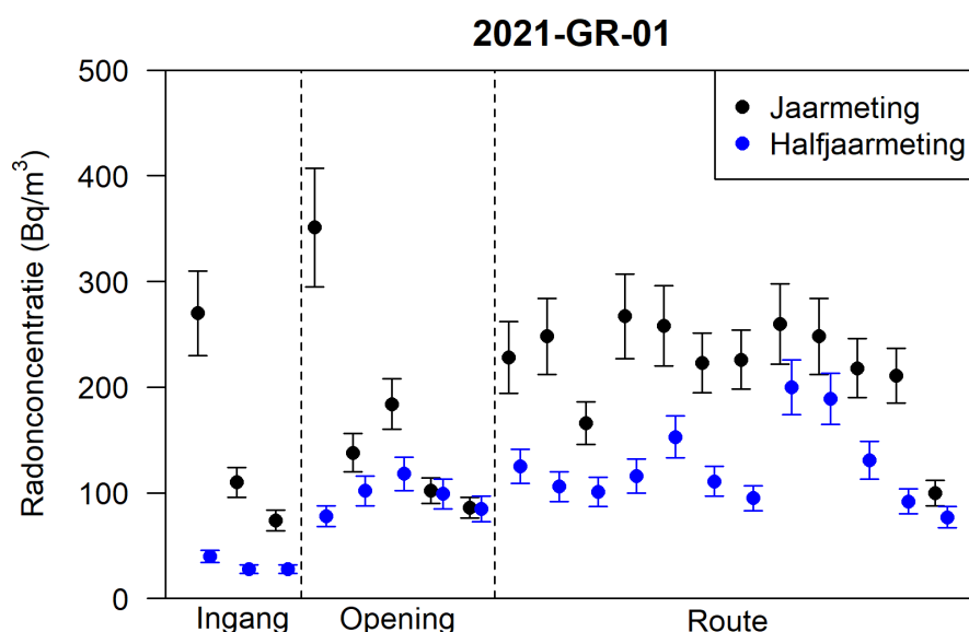
Figuur 15.1 De radonconcentratie op verschillende categorieën locaties in groeve 2021-GR-01 (zie tekst aan het begin van paragraaf 15.1 voor beschrijving).
