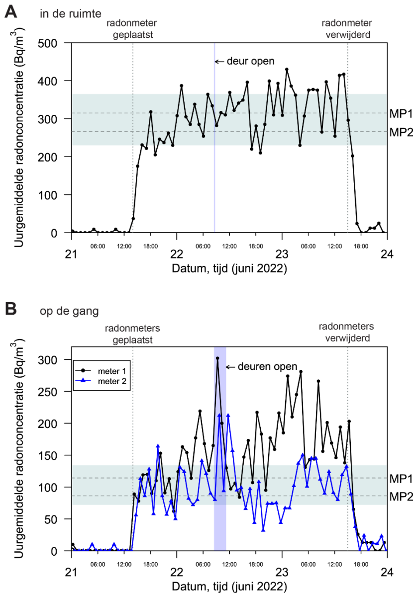
Figuur 10.2 De radonconcentratie gemeten tijdens het reinigen van de sproeikoppen in tien gecombineerde beluchtungs- en filtratieruimtes (eerste set continue metingen). Figuur A geeft de radonconcentratie in één van de ruimtes weer, en figuur B de radonconcentratie gemeten op twee verschillende locaties op de gang voor de ruimtes. Meter 1 was geplaatst aan het einde van de gang, tegenover de ruimte uit figuur A . Meter 2 was verderop in de gang geplaatst. In de periode van 08.30 tot 11.15 vond in ten minste één van de ruimtes ongeveer een kwartier lang werkzaamheden plaats, waarbij de deur van de ruimte open was. Deze tijd is gemarkeerd met een gekleurd verticaal vlak in de figuren. In de figuur is aangegeven wanneer de radonmeters zijn geplaatst en verwijderd. Daarnaast zijn twee radonconcentraties gemarkeerd: MP1 en MP2, het resultaat van passieve radonmetingen (in een vergelijkbare ruimte en op dezelfde gang) tijdens respectievelijk de eerste en tweede meetperiode. Het gekleurde horizontale vlak geeft de onzekerheid weer (2 standaarddeviaties) van de passieve metingen.
