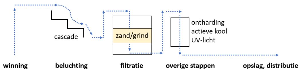
Figuur 8.2 Schematische weergave van het drinkwaterzuiveringsproces van grondwater, gebaseerd op de figuren op de websites van WML [58] en WMD Drinkwater [59]. Per waterwinningstype en productiestation is (de volgorde van) het zuiveringsproces net iets anders. Het is onder andere afhankelijk van de samenstelling van het ruwe water.
