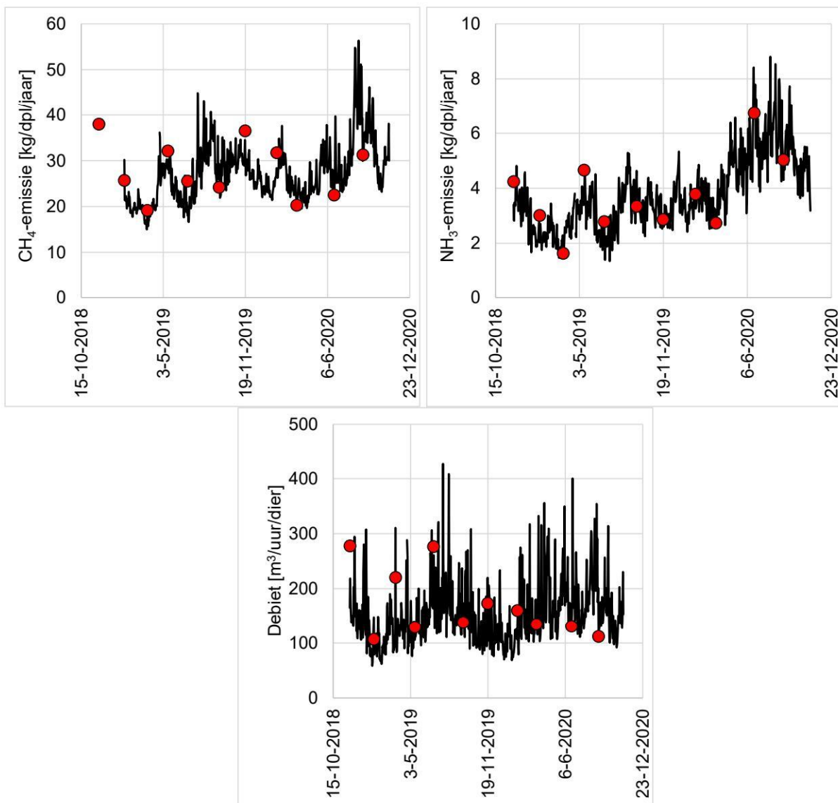
Figuur G1.4. Linksboven: CH 4 -emissie [kg/jaar per dierplaats]; Rechtsboven: NH 3 -emissie [kg/jaar per dierplaats]; Onder: Ventilatie-debiet [m 3 /uur/dier]. De protocollaire metingen worden met rode cirkels weergegeven. De emissies in deze figuur zijn niet door leegstand gecorrigeerd.
