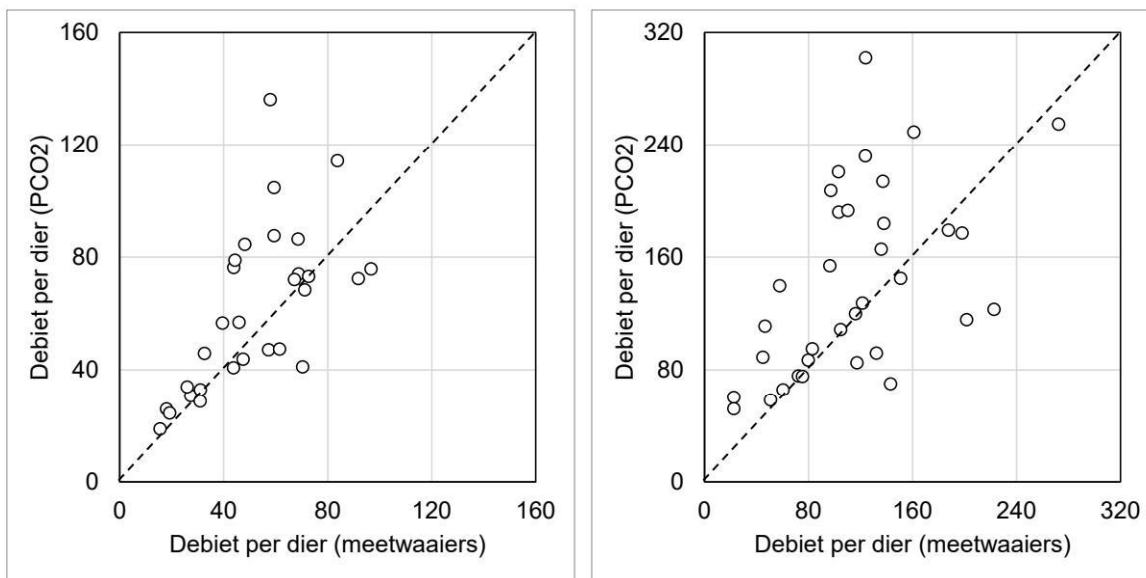
Figuur 5.2.9 Relatie tussen het ventilatiedebiet bepaald door middel van de tracergas ratiomethode (PCO 2 ) en gemeten met meetwaaiers (MV) op basis van de protocollaire metingen in rosé vleeskalverstallen. Links: opfokfase; Rechts: afmestfase.
