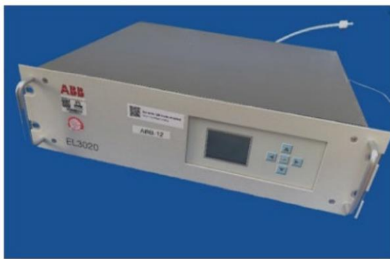
Figuur A1 Links: Dräger Polytron 8000 met de FL-6813260 sensor voor \text{NH}_3 -concentratiemetingen. Midden: Vaisala CARBOCAP® met GMP252 sensor voor \text{CO}_2 -concentratiemetingen. Rechts: ABB EasyLine EL3000 met Uras26 sensor voor \text{CH}_4 -concentratiemetingen.
