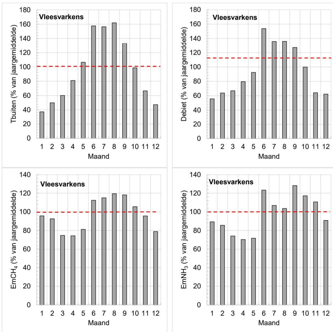
Figuur 7.2.8 Jaarpatroon voor de buitentemperatuur, het ventilatiedebiet, en de emissies van \text{CH}_4 en \text{NH}_3 , op basis van continue metingen in vleesvarkenstallen. Alle parameters zijn weergegeven als percentage van de (gemeten) jaargemiddelden (als rode stippellijn weergegeven).
