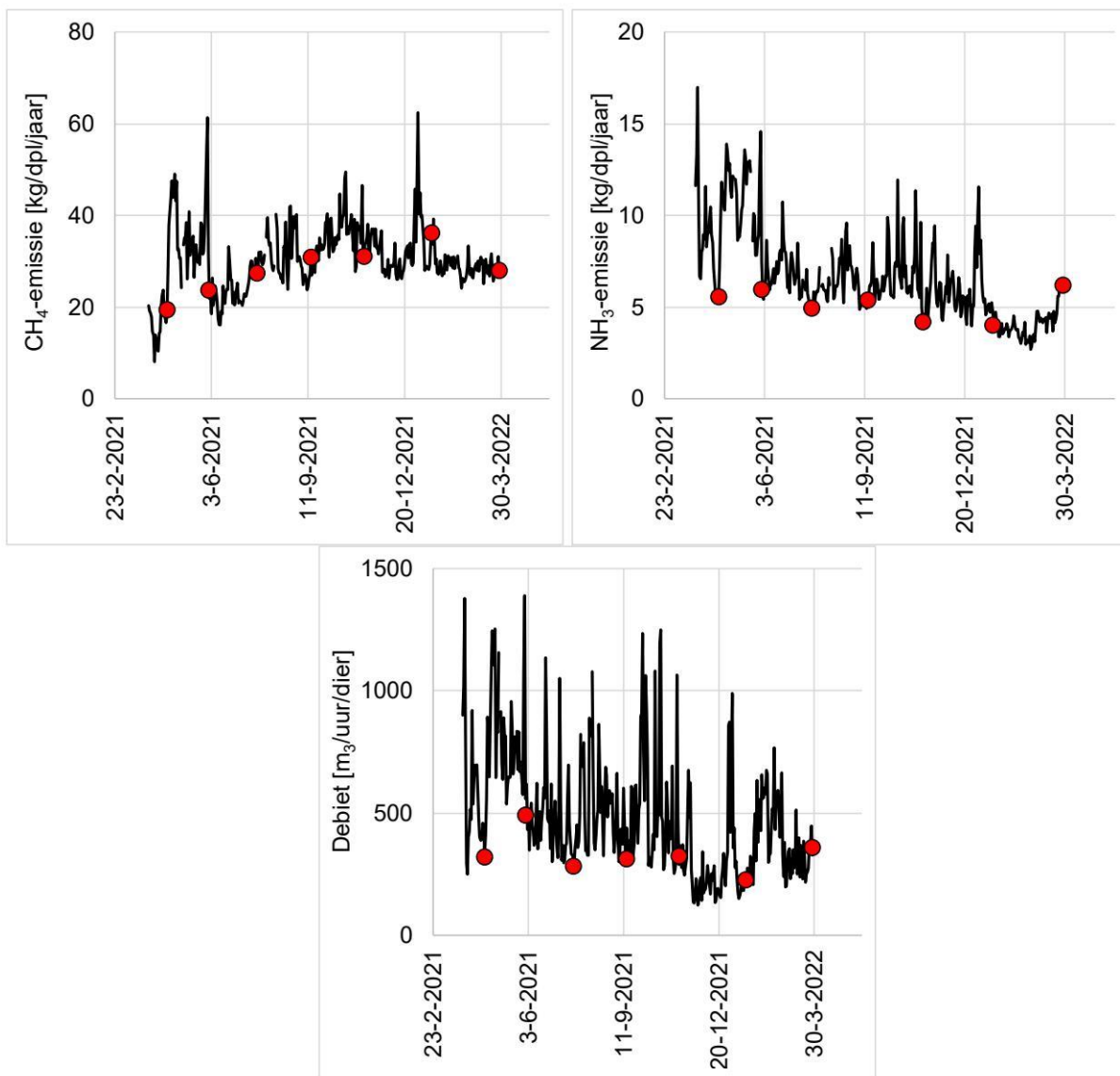
Figuur JV1.2. Linksboven: \text{CH}_4\text{-emissie [kg/jaar per dierplaats]} ; Rechtsboven: \text{NH}_3\text{-emissie [kg/jaar per dierplaats]} ; Onder: \text{Ventilatie-debiet [m}^3\text{/uur/dier]} . De protocollaire metingen worden met rode cirkels weergegeven. De emissies in deze figuur zijn niet door leegstand gecorrigeerd.
