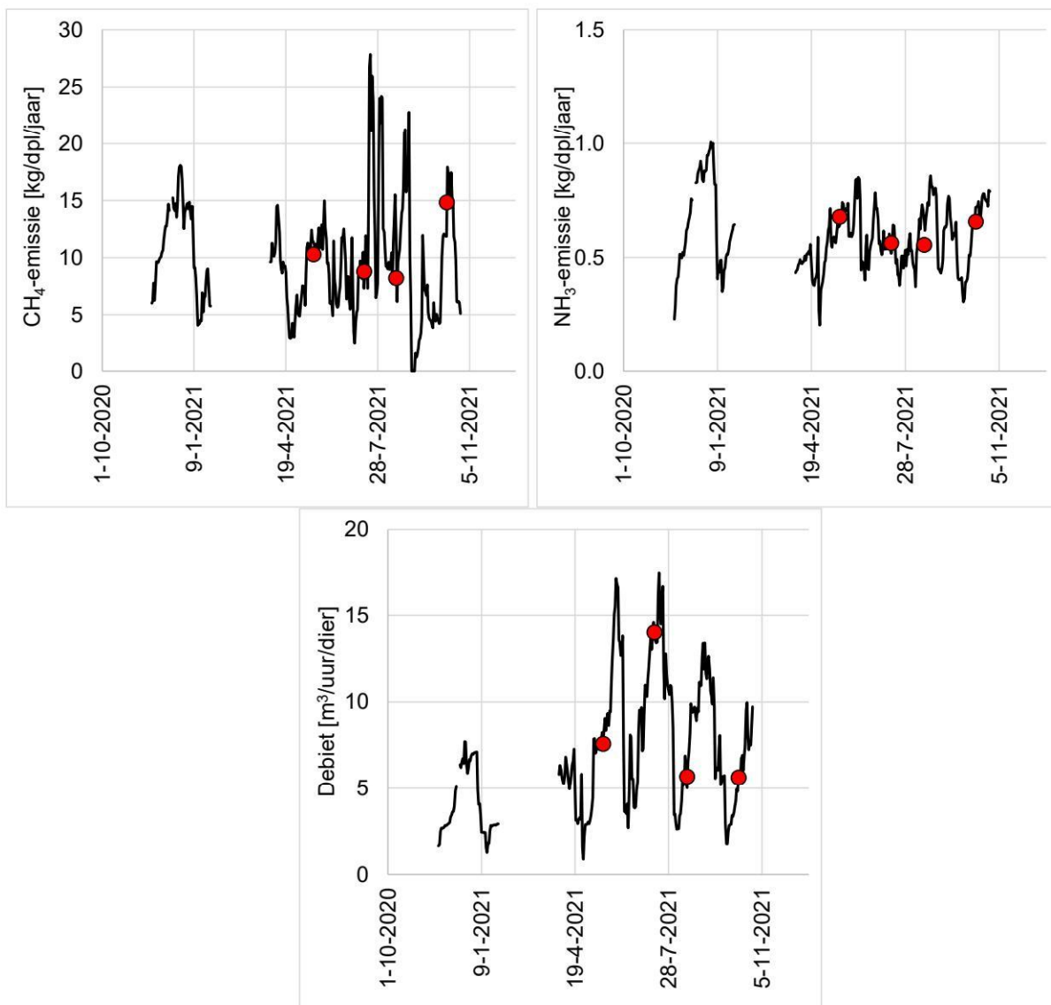
Figuur BG4.2. Linksboven: CH 4 -emissie [kg/jaar per dierplaats]; Rechtsboven: NH 3 -emissie [kg/jaar per dierplaats]; Onder: Ventilatie-debiet [m 3 /uur/dier]. De protocolaire metingen worden met rode cirkels weergegeven. De emissies in deze figuur zijn niet door leegstand gecorrigeerd.
