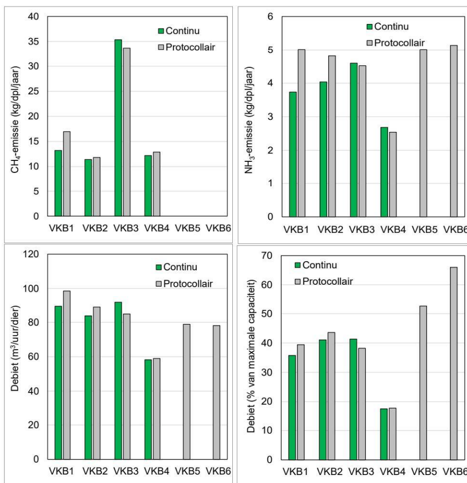
Figuur 5.1.3 Per blankveeskalverbedrijf, gemiddeld ventilatiedebiet en gemiddelde emissies van \text{NH}_3 en \text{CH}_4 voor de continue en de protocollaire metingen, wanneer gebruikt wordt gemaakt van alle beschikbare waarnemingen. Onder (rechts): per bedrijf, gemiddelde ventilatiedebiet voor de continue en de protocollaire metingen als percentage van de totale geïnstalleerde maximale ventilatiecapaciteit.
