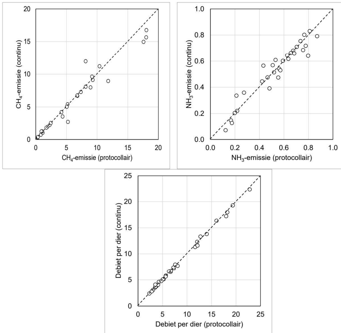
Figuur 7.1.4 Enkelvoudige lineaire regressie tussen de continue en de protocolaire metingen in biggenstallen, wanneer alleen gebruikt wordt gemaakt van de data die gemeten is tijdens de dagen waarop protocolaire metingen zijn uitgevoerd. Vergelijking is alleen voor bedrijven BG1 t/m BG4 mogelijk.
