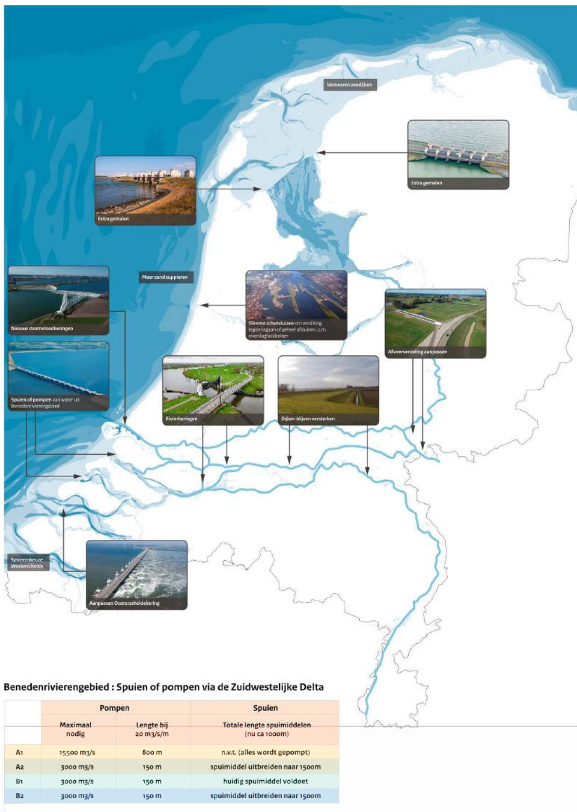
Figuur 5: De bouwstenen die nodig zijn voor het realiseren van de denkrichting Beschermen en het geschatte ruimtebeslag van benodigde pomp- dan wel spuicapaciteit.
