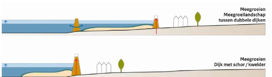
Figuur 1b: Dwarsdoorsnede van twee mogelijke bouwstenen uit de denkrichting Meegroeien. In beide gevallen zal de achterliggende dijk in de toekomst minder versterkt hoeven te worden dan zonder aanslibbing.
