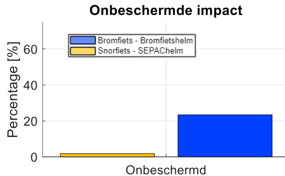
Figuur 24 Percentage van onbeschermd impacts (buiten de helm zone) voor de bromfiets met minimale bromfietshelm (bij een volledig beschermende bromfietshelm worden deze impacts dus wel opgevangen door de helm) en snorfiets met SEPAC-helm, in simulatiescenario 1.
