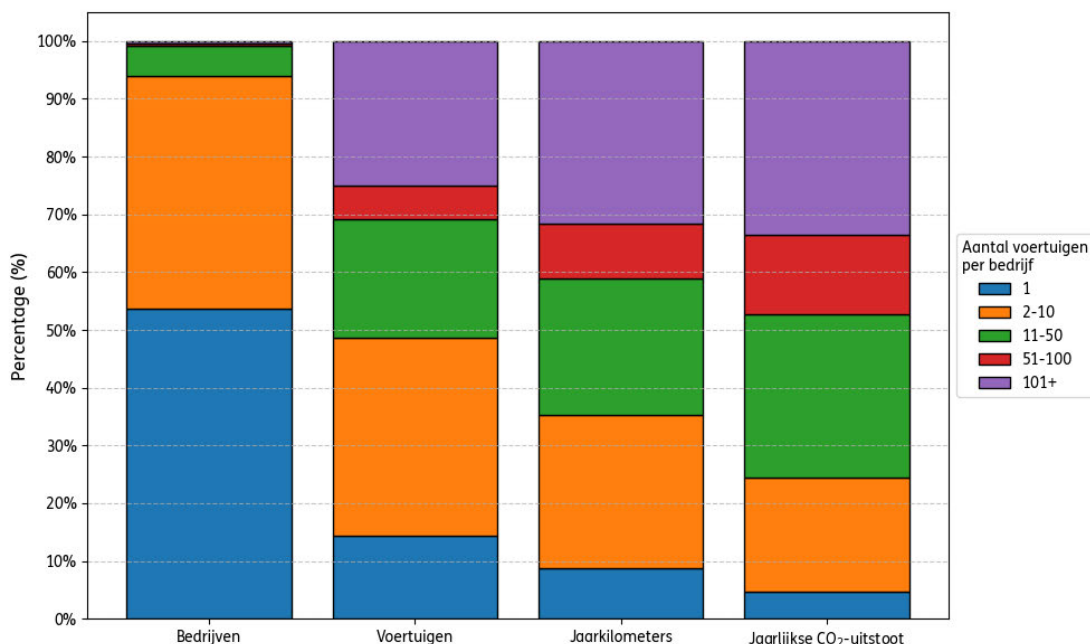
Figuur 5.4: Verdeling van bedrijven, voertuigen, kilometers en CO 2 -uitstoot per bedrijfsgrootte voor bestelauto's, vrachtauto's en trekkers samen. In de categorisatie van "Aantal voertuigen" zijn bestelauto's, vrachtauto's en trekkers meegenomen.
