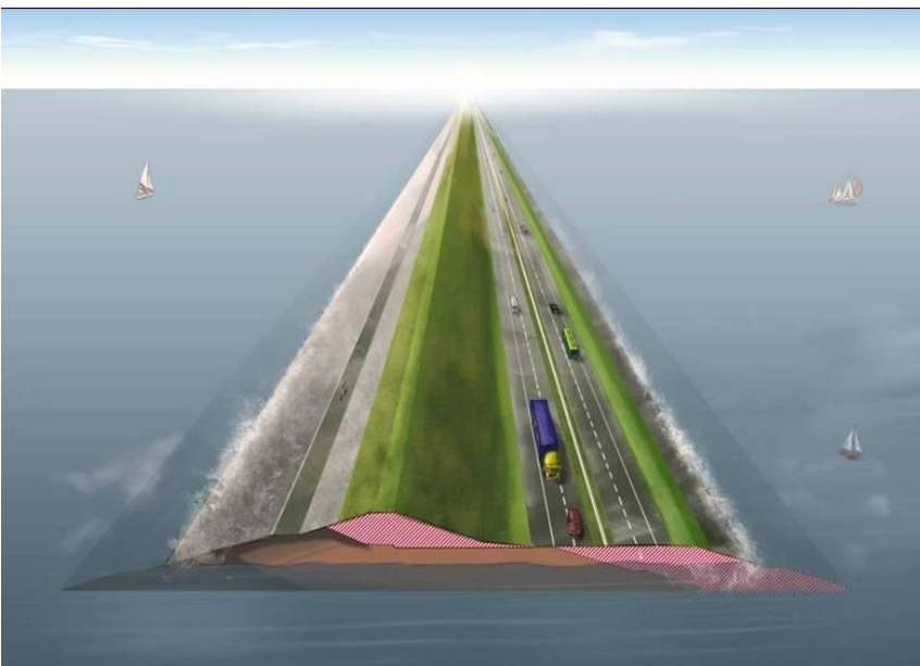
Figuur 4.2 2100-Robuust (21R): illustratie doorsnede van verhoogd en verbreed dijklichaam
