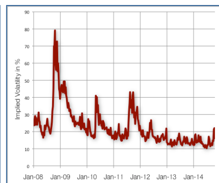
Afbeelding 4: Implied volatility
