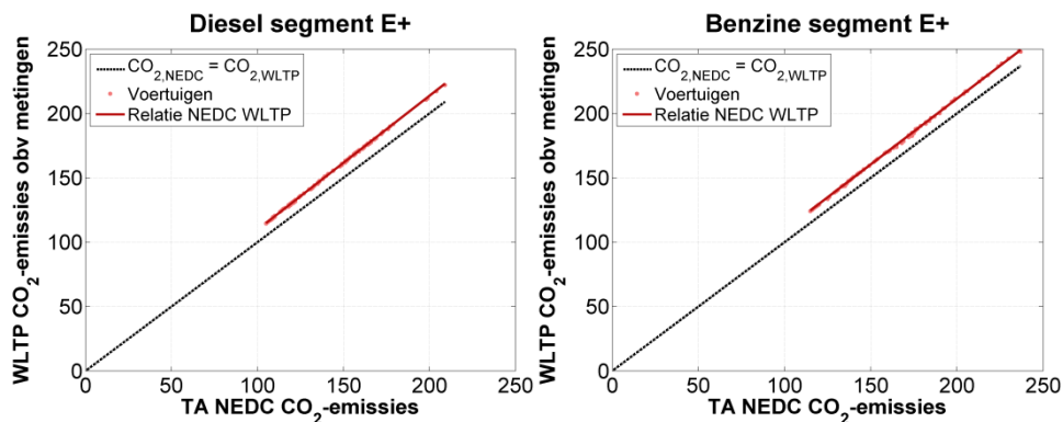
Figuur 4: NEDC CO 2 -emissies volgens typegoedkeuring en afgeleide WLTP CO 2 -emissies op basis van een correlatie afgeleid uit metingen per segment voor alle in 2015 verkochte personenautomodellen met meer dan 1000 stuks verkocht. Inclusief verkoopgewogen lineaire relaties tussen de NEDC en WLTP emissies.
