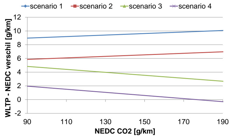
Figuur 10: Diesel - verschil WLTP-NEDC voor scenario's S1-S4 voor 2018
