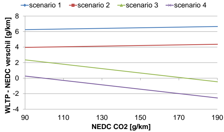
Figuur 9: Benzine - verschil WLTP-NEDC voor scenario's S1-S4 voor 2018
