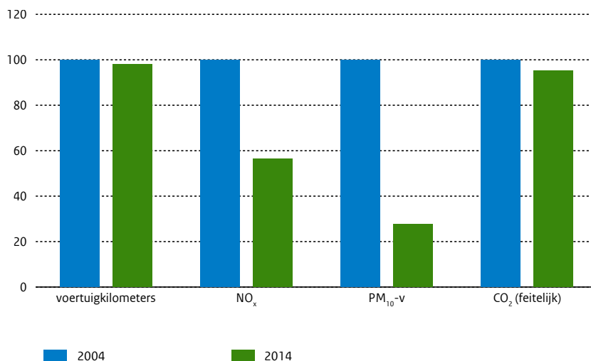
Figuur 1 Ontwikkeling voertuigkilometers en emissies van NO x , verbrandingsfijnstof (PM 10 -v) en CO 2 feitelijk van het totale vrachtautopark (inclusief trekkers). Bron: Emissieregistratie (2015).
