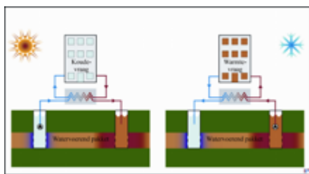
Figuur 9. Schematische weergave van open en gesloten bodemenergiesystemen
