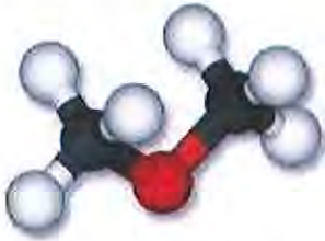
Figuur 7 DME molecuul. Twee koolstofatomen (zwart), één zuurstof atoom (rood) en zes waterstofatomen (wit).
