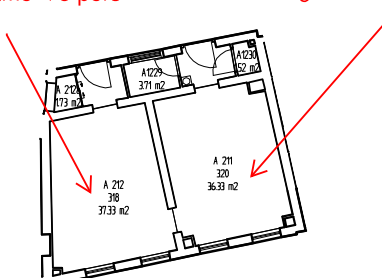
Tweede verdieping
