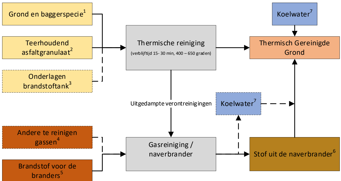
Figuur 2.2 Schematisch overzicht van het thermische reinigingsproces van verontreinigde grond. Gestippelde boxen en lijnen geven aan dat deze handeling producent specifiek is. Hierna volgt een toelichting op enkele textboxen.
