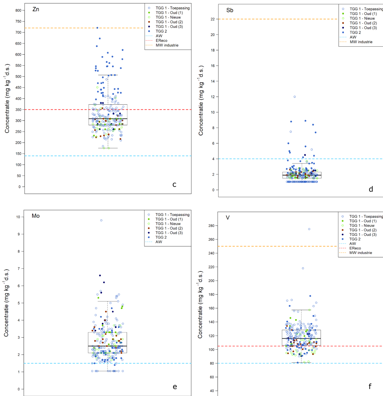
Figuren 4.2 a t/m e Verdeling van concentraties arseen* (a), koper (b), zink (c), antimoon* (d), molybdeen* (e) en vanadium** (f) in TGG zowel depot als praktijkcasus Bunschoten. De concentraties zijn omgerekend naar een standaard bodem. De blauwe lijn geeft de AW weer, de gele lijn de MW I en de rode het Ernstig risico niveau voor ecologie (ER eco ).
