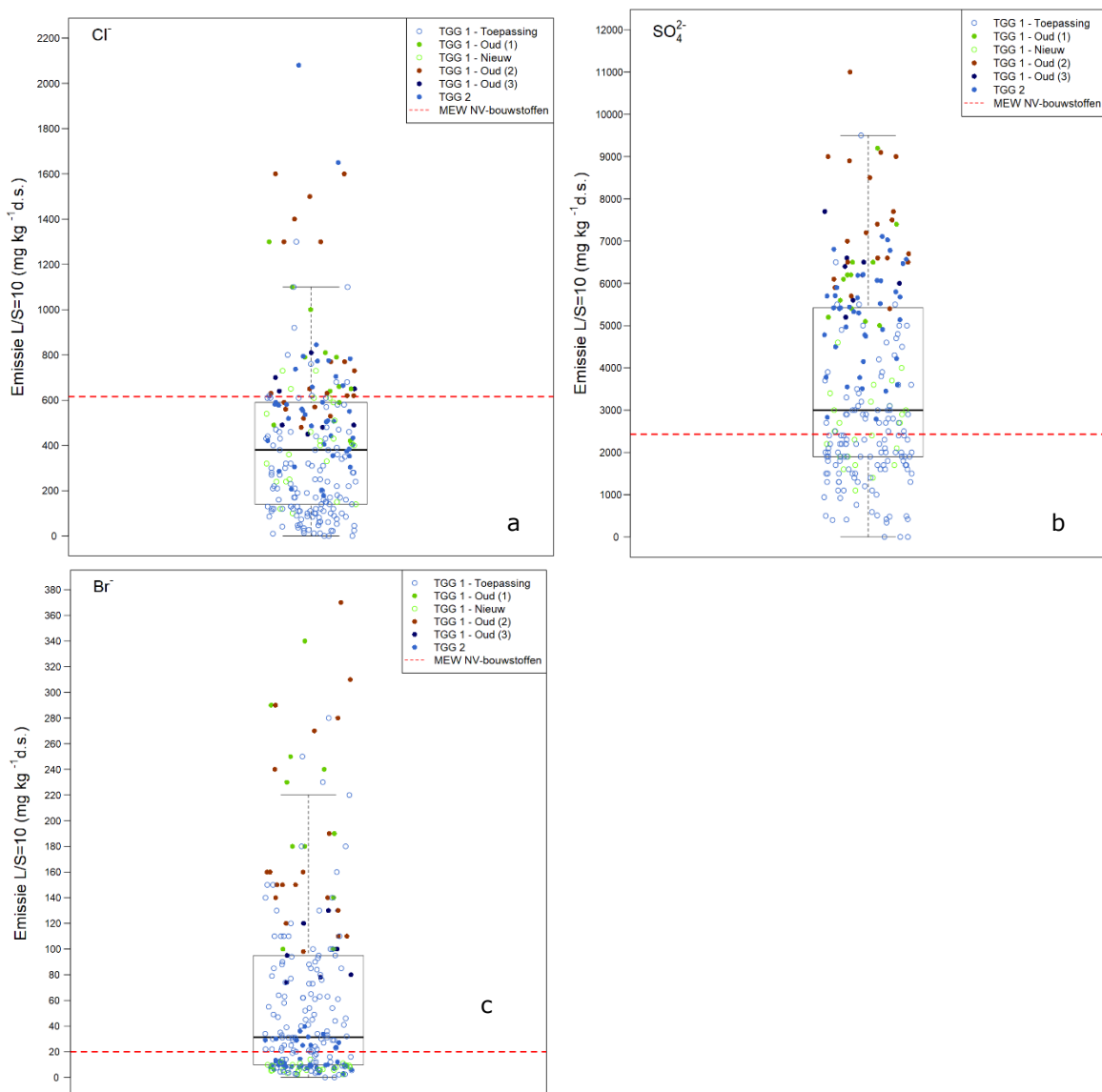
Figuur 4.5 a t/m c uitloogconcentraties (mg kg -1 L/S10) Chloride (a), sulfaat (b) en bromide (c) uit TGG in depot. De rode lijn vertegenwoordigt de Maximale emissiewaarde voor niet-vormgegeven bouwstoffen.
