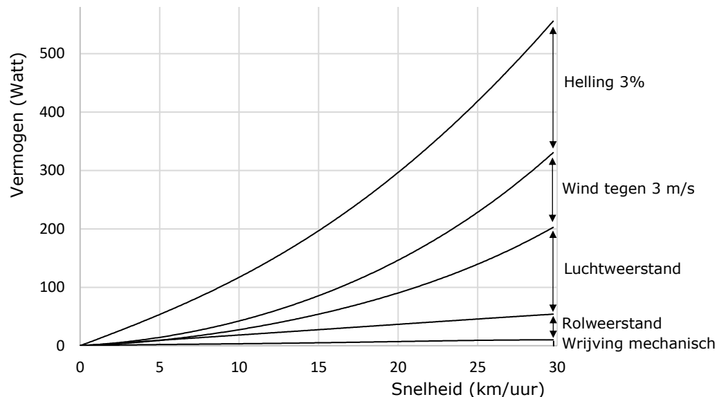
Afbeelding 8. Door een fietser te leveren uitwendig vermogen om de verschillende tegenkrachten te overwinnen, afhankelijk van de rijnsnelheid (CROW, 1993; Van Laarhoven & Ploeger, 1980)
