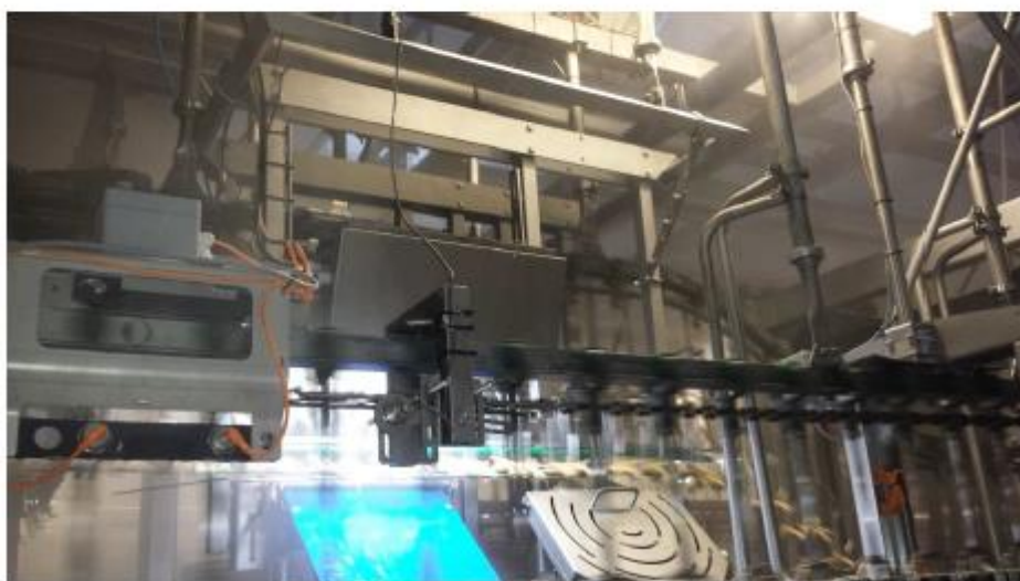
Figuur 21: camera set-up van het Meyn Footpad Inspection System in het slachthuis uit Van Harn & De Jong (2017).
