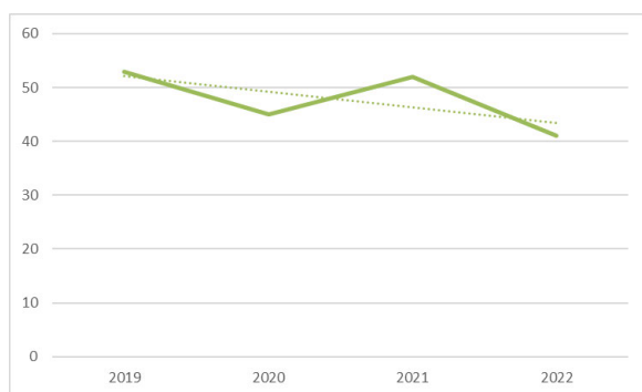
Figuur 1819 Spoorstaafbreuken 2019-2022
