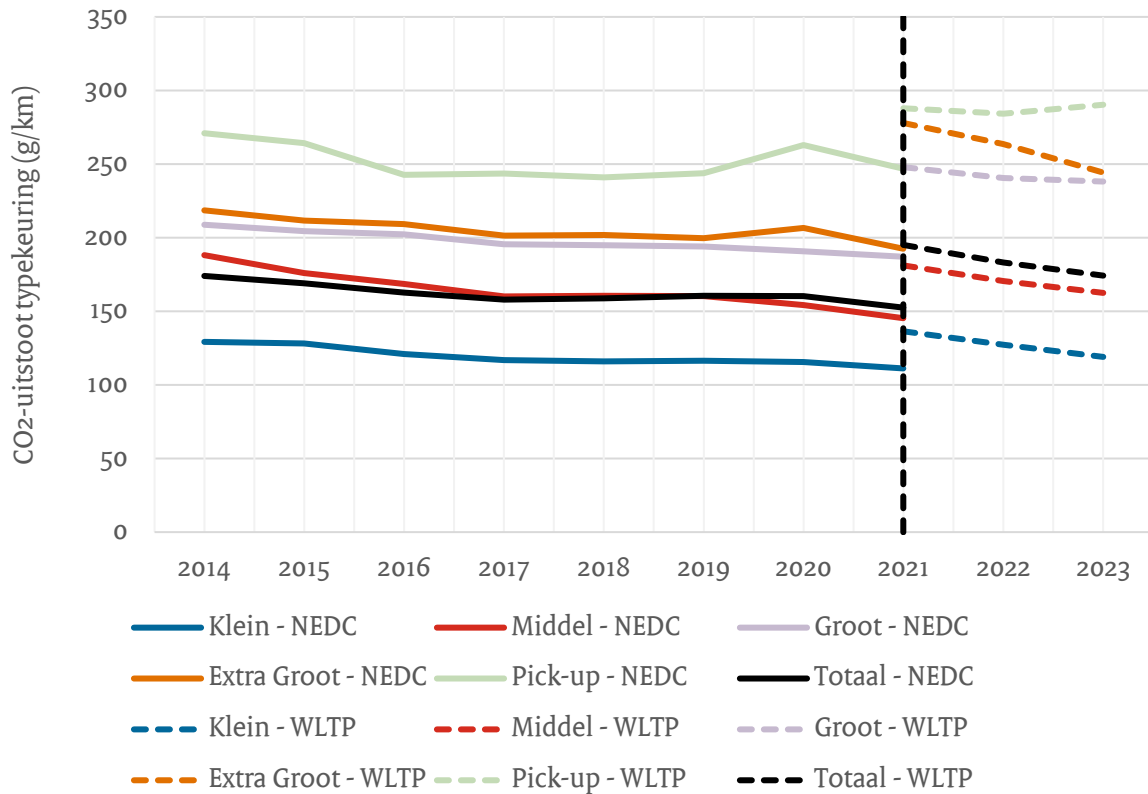
Figuur 14: Gemiddelde CO 2 -uitstoot (NEDC/WLTP) per segment, nieuwverkopende aandrijflijnen jaar ultimo 2014-2022 en 2023 t/m juni
