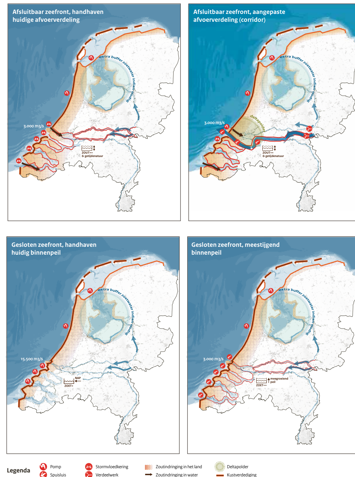
Figuur 4: De onderzochte 4 strategieën van de denkrichting Beschermen: afsluitbaar zeefront met stormvloedkeringen, meestijgend waterpeil en al dan niet aangepaste afvoer-verdeling Rijntakken. En gesloten zeefront met hetzij pompen en een laag waterpeil, of spuien en een meestijgend waterpeil om overtollig rivierwater naar zee af te voeren. Door de verschillende combinaties van bouwstenen verschillen de strategieën in optredende verzilting en benodigde dijkversterkingen.
