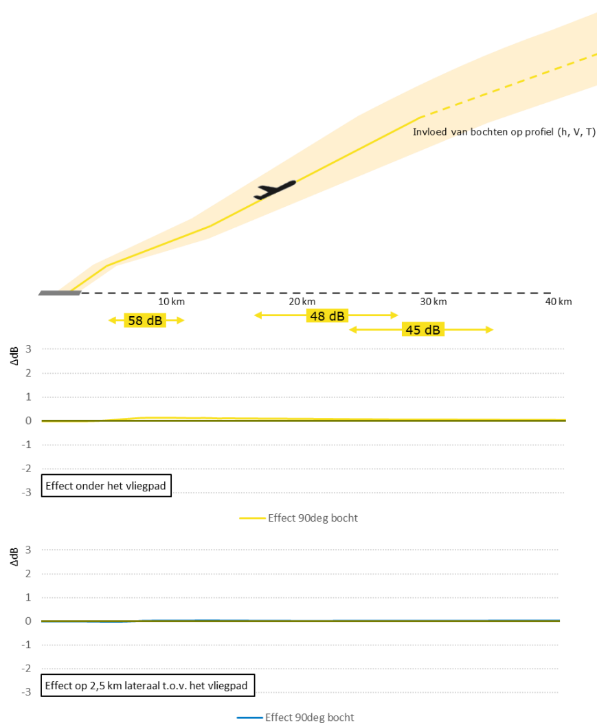
Figuur 0-11 Geluideffecten als gevolg van de invloed van een bocht, ten opzichte van de standaard aanname dat bochten geen invloed hebben op de vliegprestaties.
