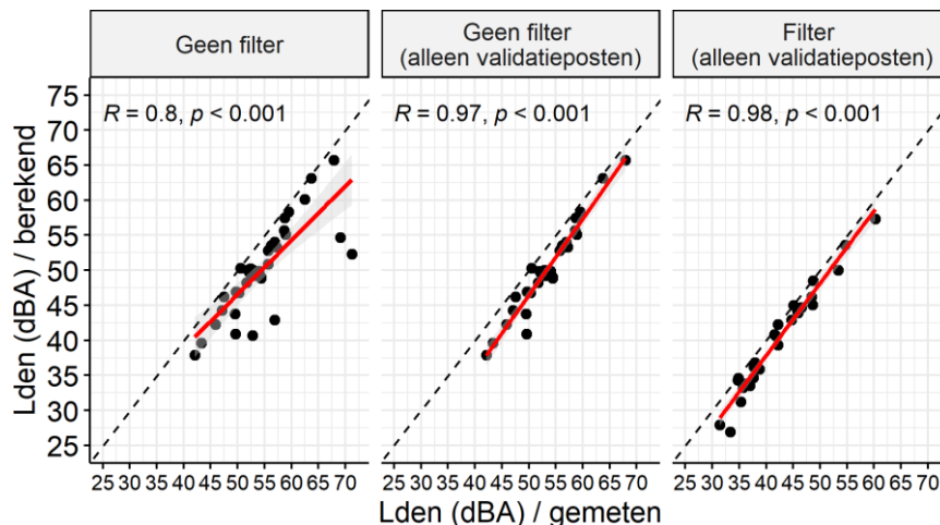
Figuur 33 Correlatie tussen gemeten en berekende geluidbelasting – zonder toepassing van validatiefilters op alle meetposten (links), alleen voor validatie meetposten (midden) en na het toepassen van validatiefilters op validatie meetposten (rechts)
