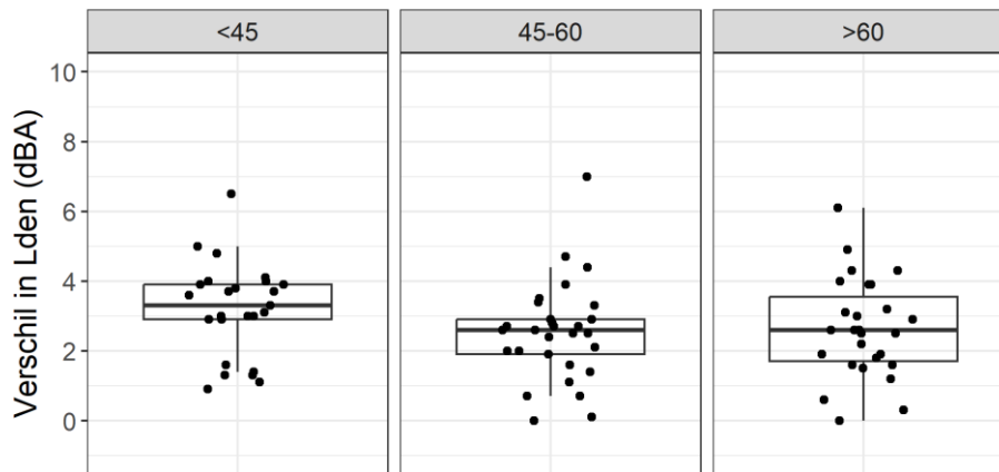
Figuur 30 Effect van elevatiehoek op het verschil tussen gemeten en berekende geluidbelasting
