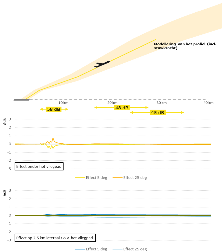
Figuur 0-8: Geluidseffekten als gevolg van de invloed van een lagere en hogere temperatuur op de vliegprestaties, ten opzichte van de standaardtemperatuur van 15 graden.
