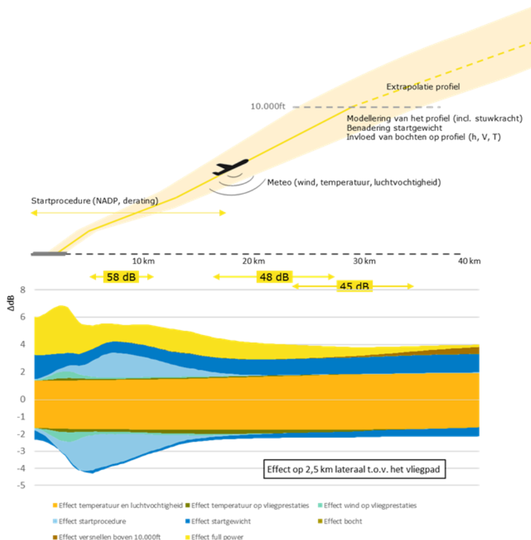
Figuur 2 Gezamenlijk effect van diverse invoerparameters voor starts op 2,5 km lateraal ten opzichte van het vliegpad
