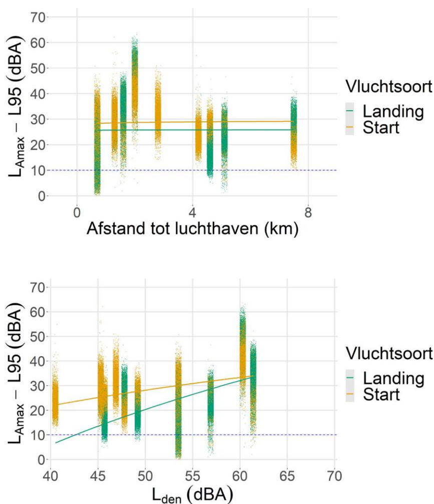
Figuur 26 Verskil tussen L_{Amax} en L_{95} per meetpost voor Eindhoven Airport met opsplitsing op basis van vluchtsoort – als functie van afstand tot de luchthaven (boven) en als functie van geluidbelasting (onder)
