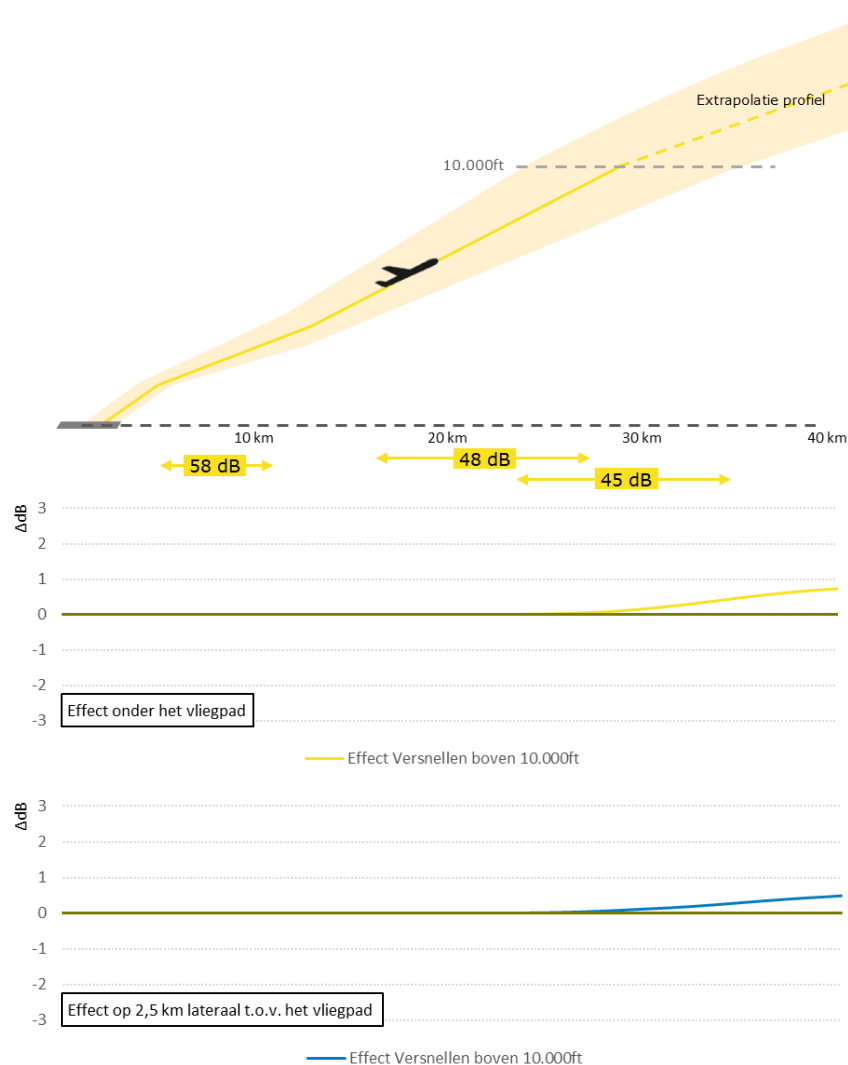
Figuur 0-10 Geluideffecten als gevolg van de alternatieve verlenging voor het simuleren van het effect van een versnelling boven een hoogte van 10.000 voet.
