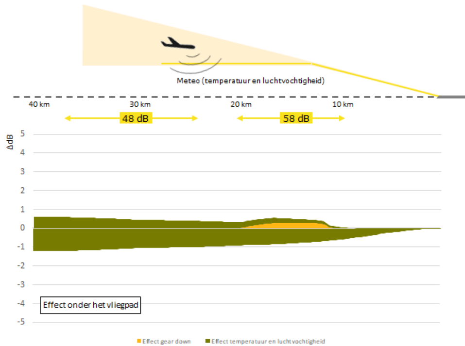
Figuur 3 Gezamenlijk effect van diverse invoerparameters voor landingen onder het vliegpad
