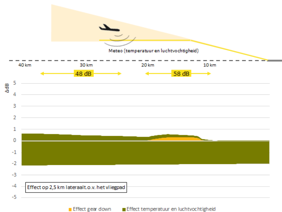
Figuur 4 Gezamenlijk effect van diverse invoerparameters voor landingen op 2,5 km lateraal ten opzichte van het vliegpad
