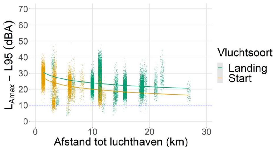
Figuur 14 Het verschil tussen L_{Amax} en L95 per meetpost voor Schiphol als functie van afstand tot de luchthaven met opsplitsing op basis van vluchtsoort
