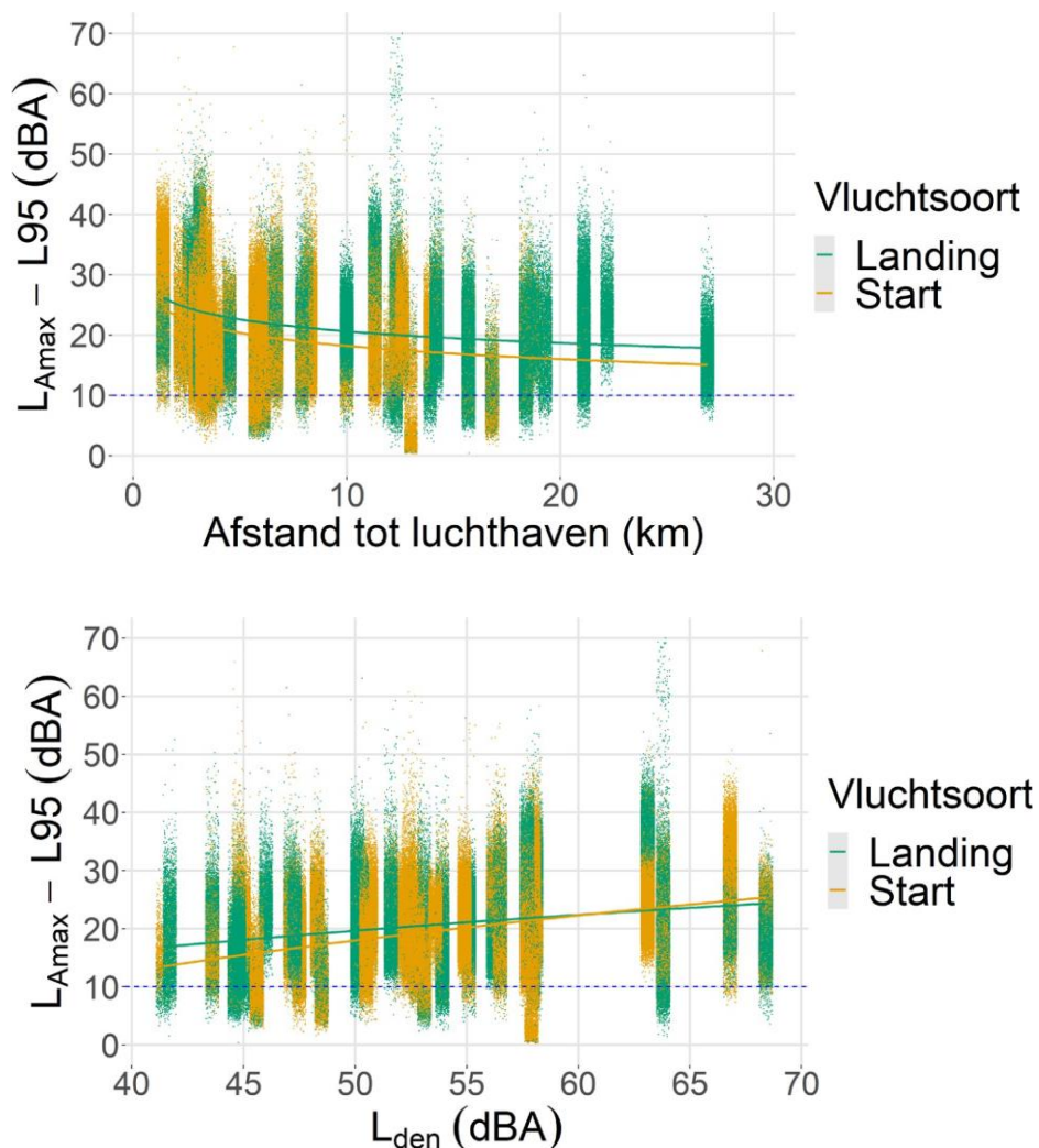
Figuur 21 Het verschil tussen L_{Amax} en L_{95} per meetpost voor Schiphol met opsplitsing op basis van type vlucht – als functie van afstand tot de luchthaven (boven) en als functie van geluidbelasting (onder)
