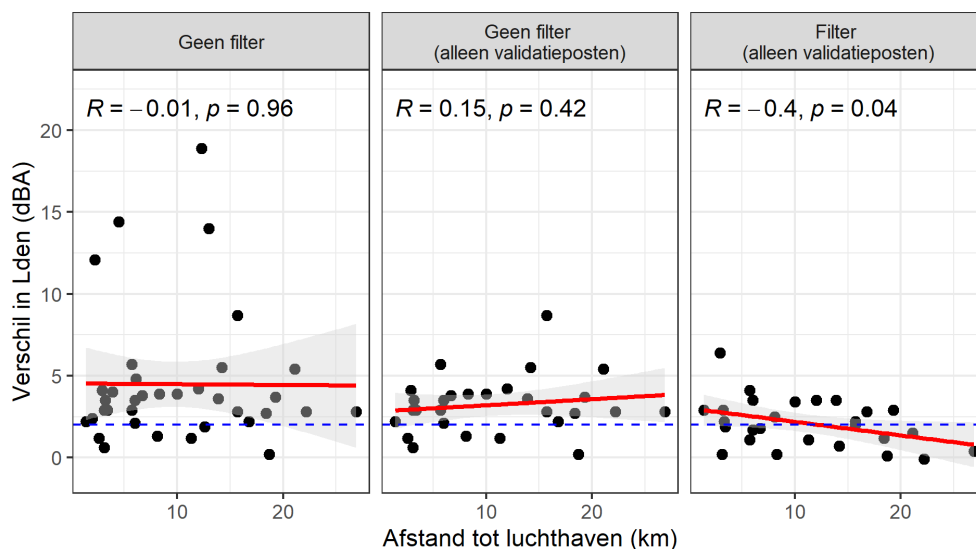
Figuur 35 Verschil tussen gemeten en berekende geluidbelasting als functie van afstand tot de luchthaven – voor alle meetposten zonder validatie-filters toegepast (links), voor alleen validatie meetposten zonder filters toegepast (midden) en voor alleen validatie meetposten met filters toegepast (rechts)
