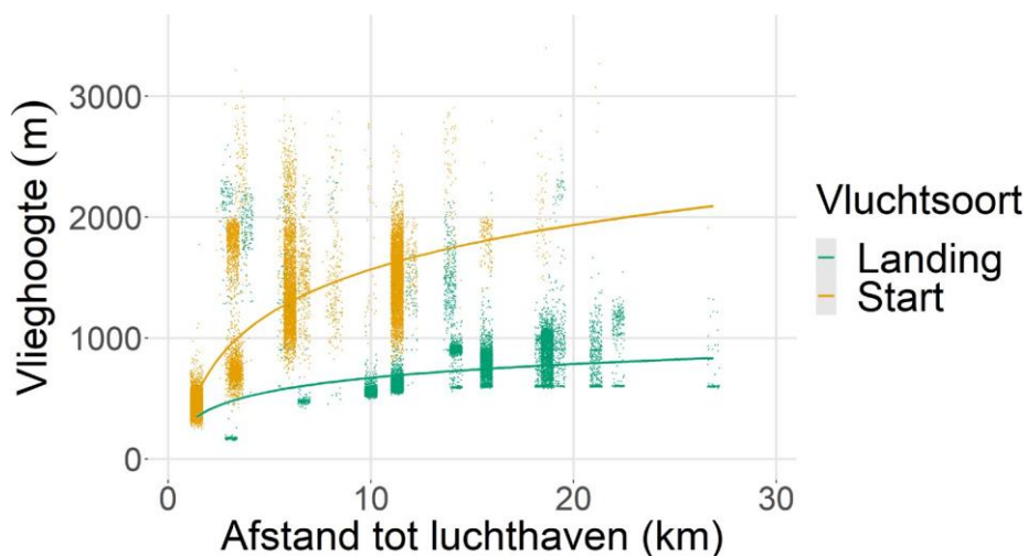
Figuur 16 Verloop van vlieghoogte voor zowel starts als landingen op de NOMOS-metposten als functie van afstand tot de luchthaven
