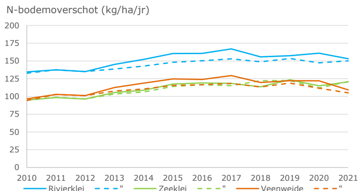
Figuur 3.7b Berekend verloop van het N-bodemoverschot (kg/ha/jr.) van landbouwgronden in de Rivierklei, de Zeeklei- en de Veenregio. Getrokken lijnen geven de situatie weer bij plaatsing van 'te plaatsen dierlijke mest' en stippellijnen geven de situatie weer bij bemesting binnen de gebruiksruimte.
