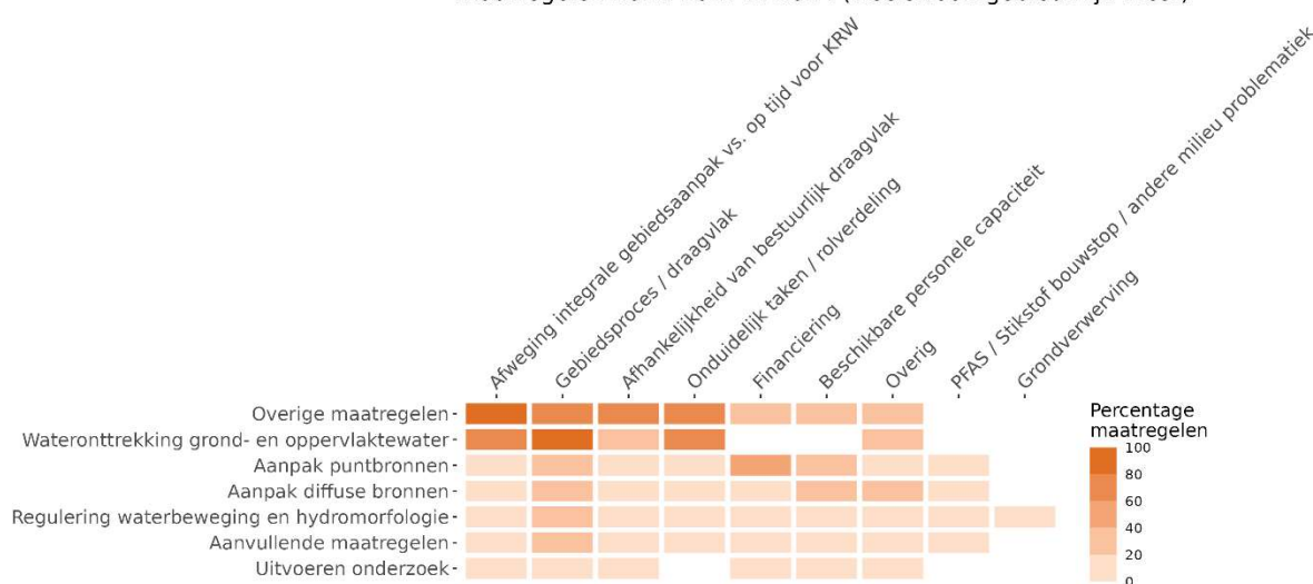
Percentage verschillende risico's benoemd voor niet tijdige uitvoering van maatregelen 2022-2027 in 2024 (Deelstroomgebied Rijn-West)
