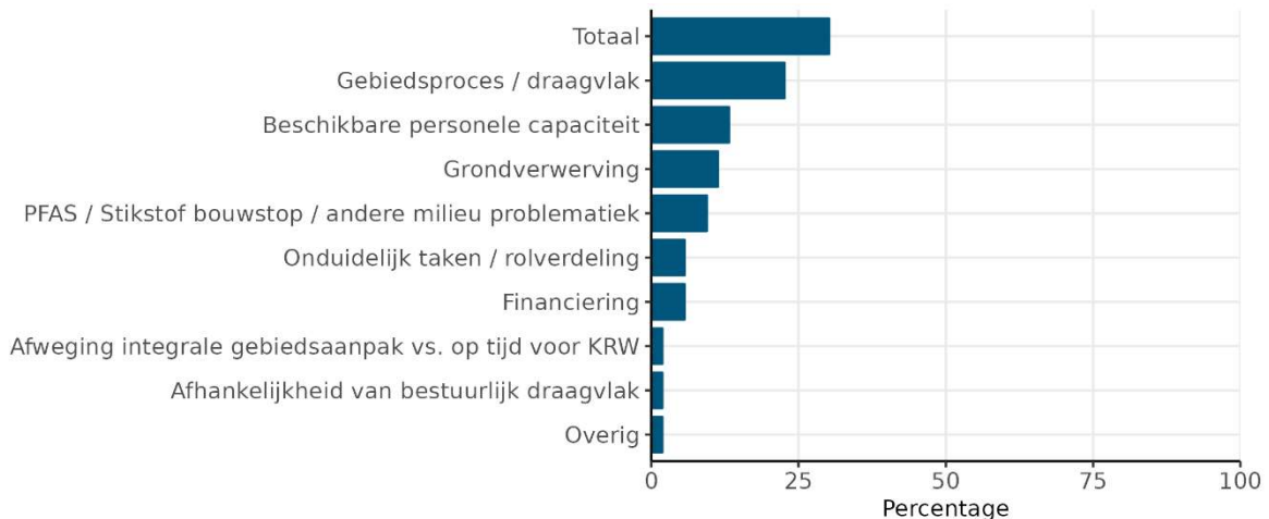
Figuur 24 Percentage gebiedsgerichte maatregelen in deelstroomgebied Schelde met een risico op niet-tijdige uitvoering. Daarbij is een nadere onderverdeling gemaakt naar de (meest) gerapporteerde risico categorieën.
