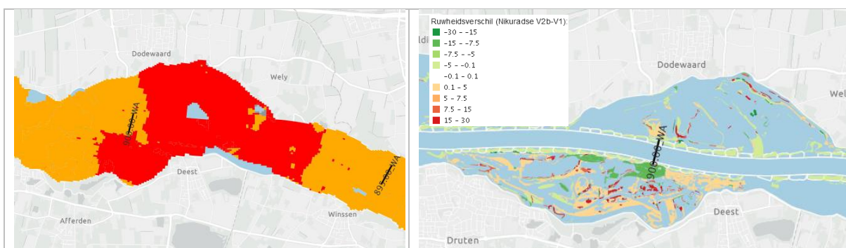
Figuur 46. Waterstandsverschil Waal km 906, ongesaldeerd (V2a vs V1) (links) en ruwheidsverschil (rechts).
