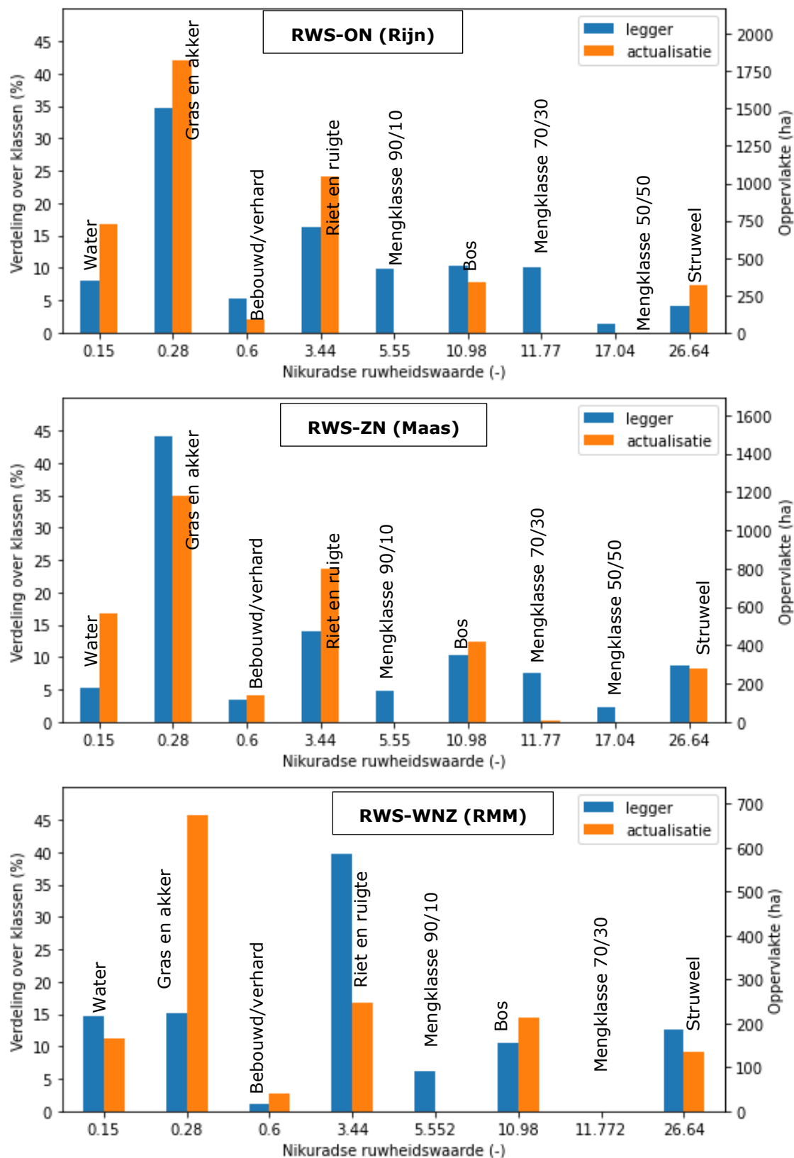
Figuur 19. De ruwheidsverdeling bij RWS-ON (Rijn, boven), RWS-ZN (Maas, midden) en RWS-WNZ (Rijn-Maas Monding, onder) voor de actuele situatie (variant V2b, gesaldeerd; variant V5 voor RMM) en de legger (variant V1). Let op dat enkel de veranderde vegetatie-oppervlaktes hierin zijn meegenomen. Het totale oppervlakte (100%) komt hierdoor overeen met de totale oppervlakte aan veranderde vegetatie in de uiterwaarden.
