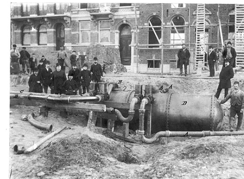
DISTRICT RESERVOIR XXXX IN DE ROEMER VISSCHERSTRAAT. A. HOUTBOUW. B. CENTRALE LUCHTBUS. C. CENTRALE TRANSPORTBUS. D. RESERVOIR RINGEN DIJK 12079.
