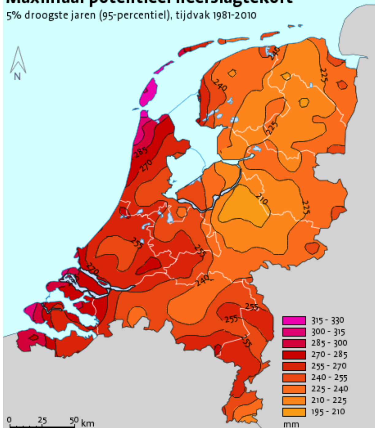
Figuur 1.31 en 1.32: potentieel neerslagtekort mediaan 1981 -2010 (links) en Maximaal potentieel neerslagtekort over de 5% droogste jaren (rechts.) Bron: KNMI, 2010.
