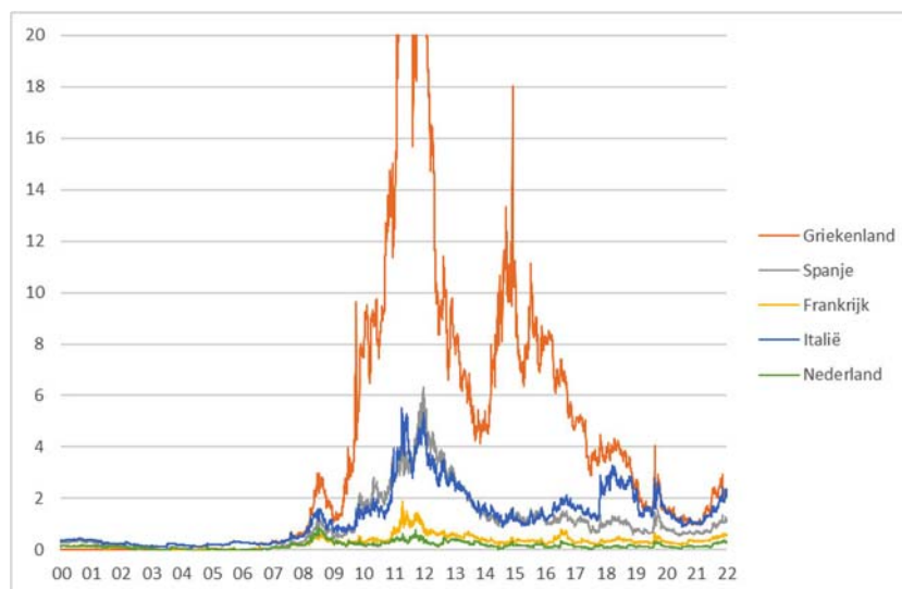
Figuur 3: De 10-jaars rentespreads (verschil met de Duitse rente)
