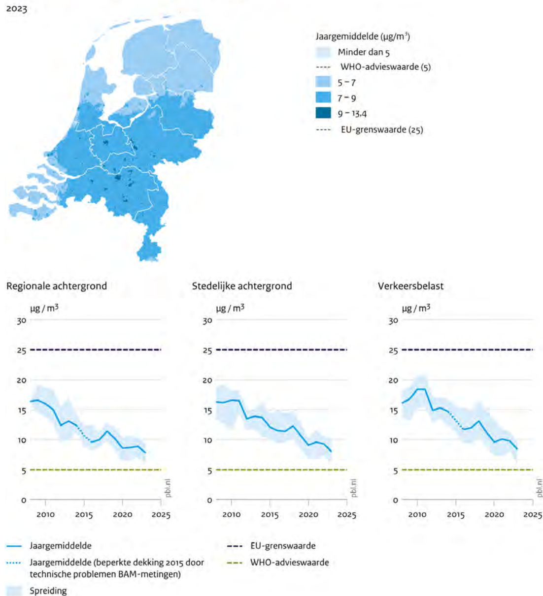
Figuur 3.26 Concentratie fijnere fractie van fijnstof (PM 2,5 ) in lucht
